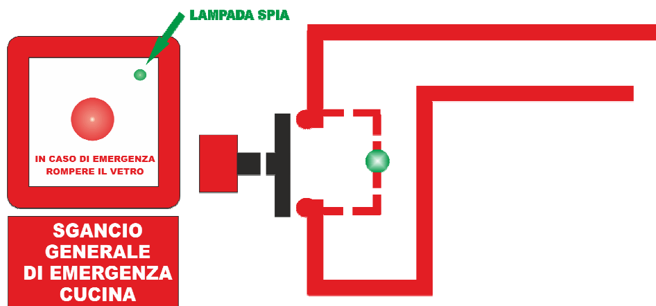
Fig. 8.1.3– Schema del circuito dello sgancio di emergenza con spia per il controllo dell'integrità del circuito
