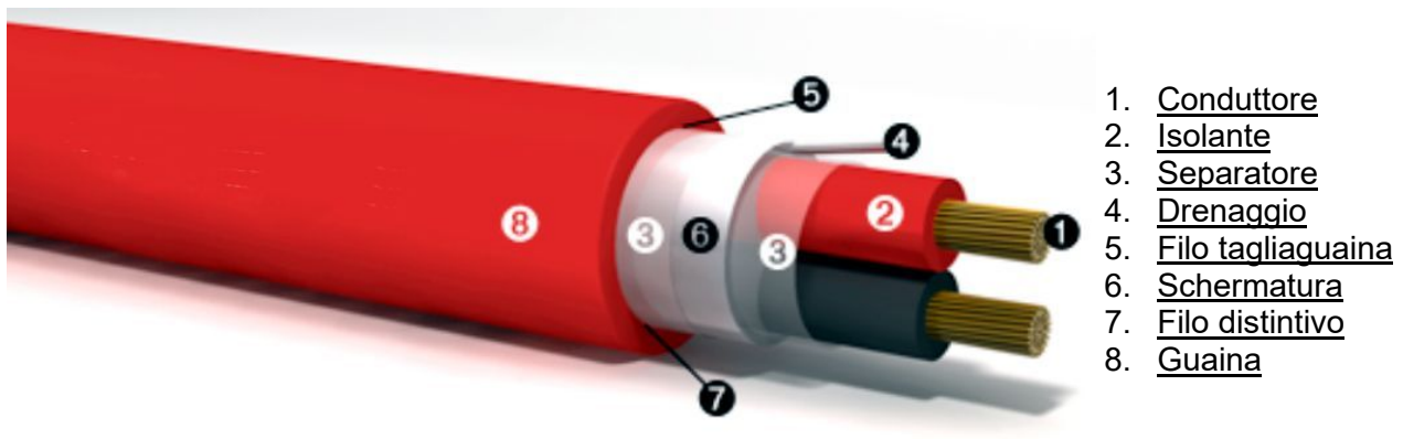
Fig. 14.3.1 - Cavi elettrici per applicazioni in sistemi fissi automatici di rivelazione e di segnalazione allarme incendio resistenti al fuoco, non propaganti l'incendio, senza alogeni.
