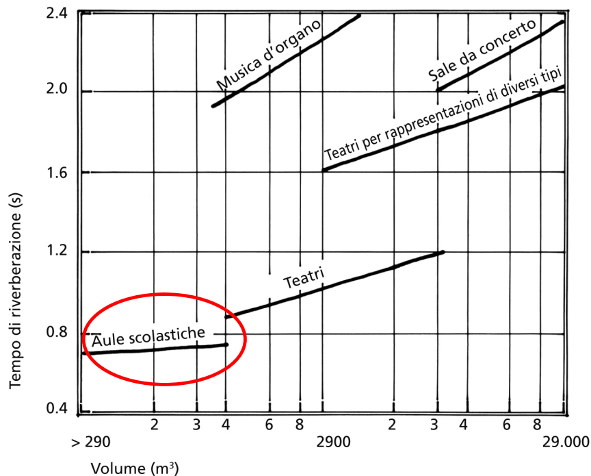
Tempi di riverberazione ottimali per le diverse destinazioni d'uso.
