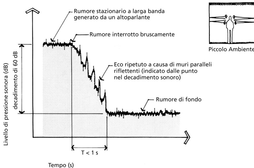
Tempo di riverberazione in un ambiente grande e piccolo.
