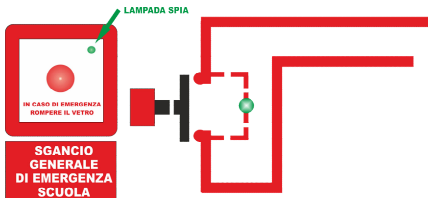
Fig. 8.1.2 – Schema del circuito dello sgancio di emergenza con spia per il controllo dell'integrità del circuito
