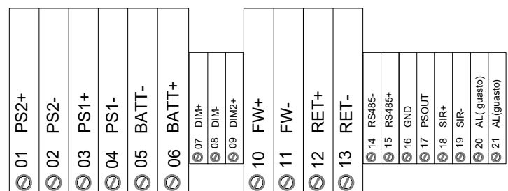
CONNETTORE su SCHEDA TD571
