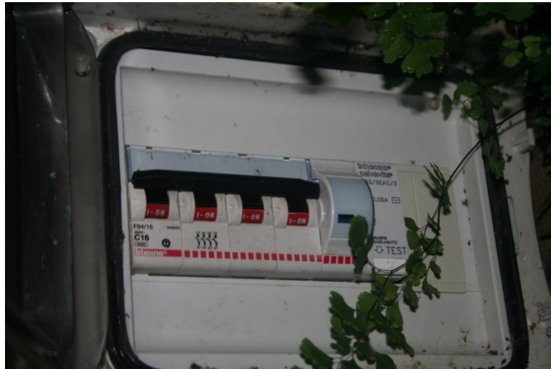
Fig. 3.3.1 – quadro elettrico generale esterno centrale termica.
