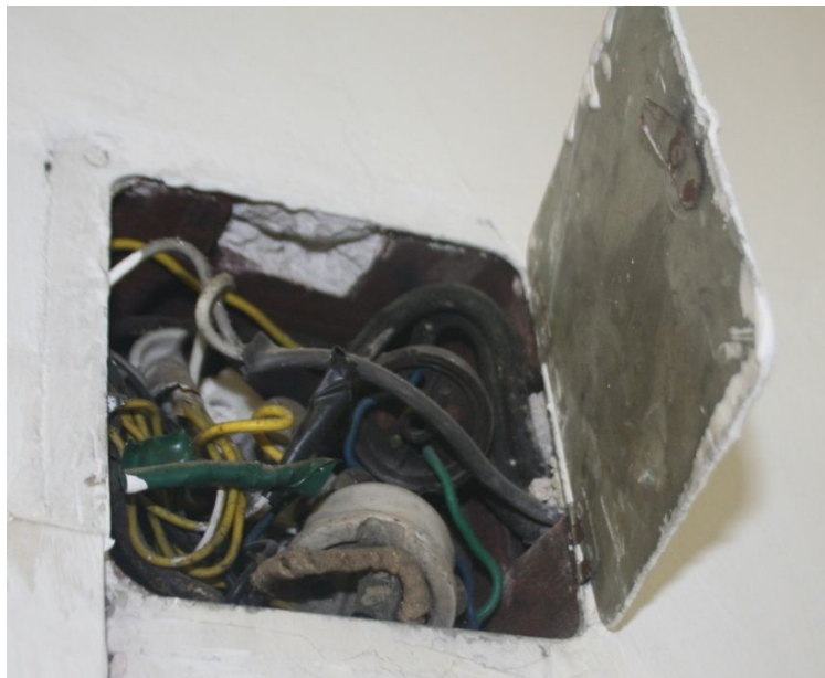
Fig. 3.2.1 – Cassetto di derivazione del vecchio impianto incassato, non sono rispettati i codici dei colori, non vi è il conduttore di terra e le giunzioni sono fatte col nastro adesivo.
