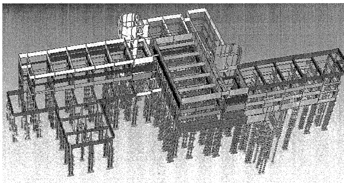
MODELLO AGLI ELEMENTI FINITI COMPLESSO SCOLASTICO CA' DI VENTURA (3900 nodi, 3000 elementi trave, 1000 elementi piastra, 2250 vincoli)
