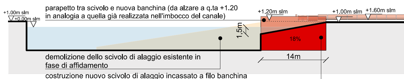
Sezione schematica andamento scivolo_ scala 1:500
