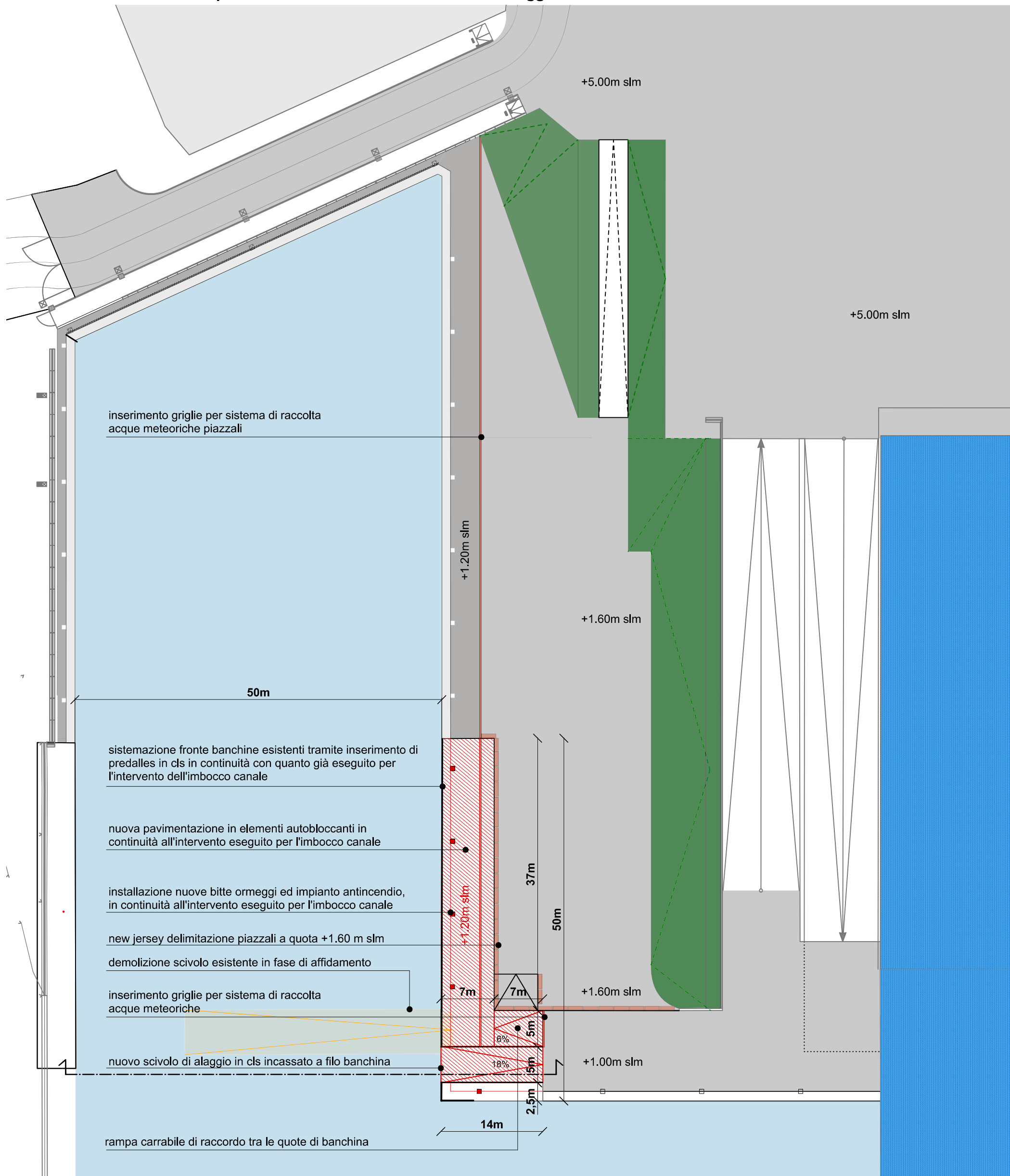
Planimetria con indicazione delle opere da realizzare in continuità all'intervento eseguito per l'imbocco canale_ scala 1:500
