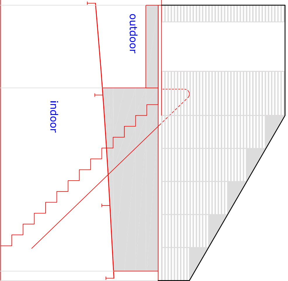
VISTA A-A
