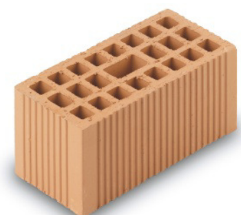
Figura 19.2 - Esempio di mattone semipieno 15\% < \Phi \leq 45\% in laterizio per murature portanti
