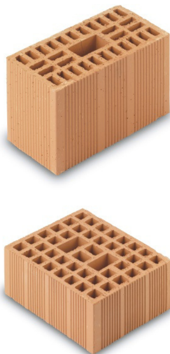
Figura 19.4 - Esempi di blocchi forati 45\% < \Phi \leq 55\% in laterizio per murature portanti
