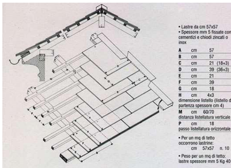
Figura 2- Dettaglio copertura tradizionale tipo in abbadini d' ardesia
