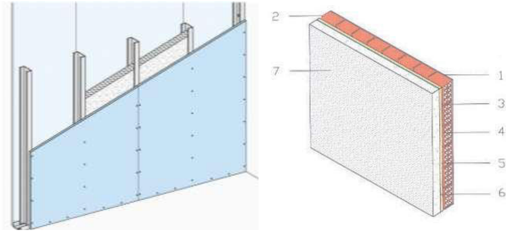
Figura 8 - Tipologie di pareti interne
