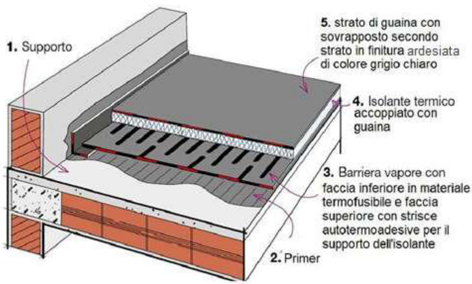
Figura 1 - Stratigrafia tipo di una copertura piana
