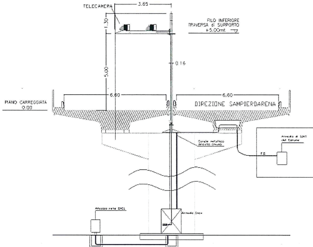
Figura 1 – Nuovo Portale ad "L"
