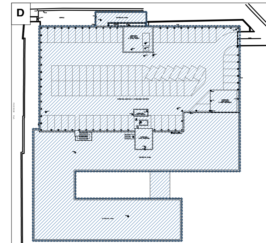
-PIANTA COPERTURA-
