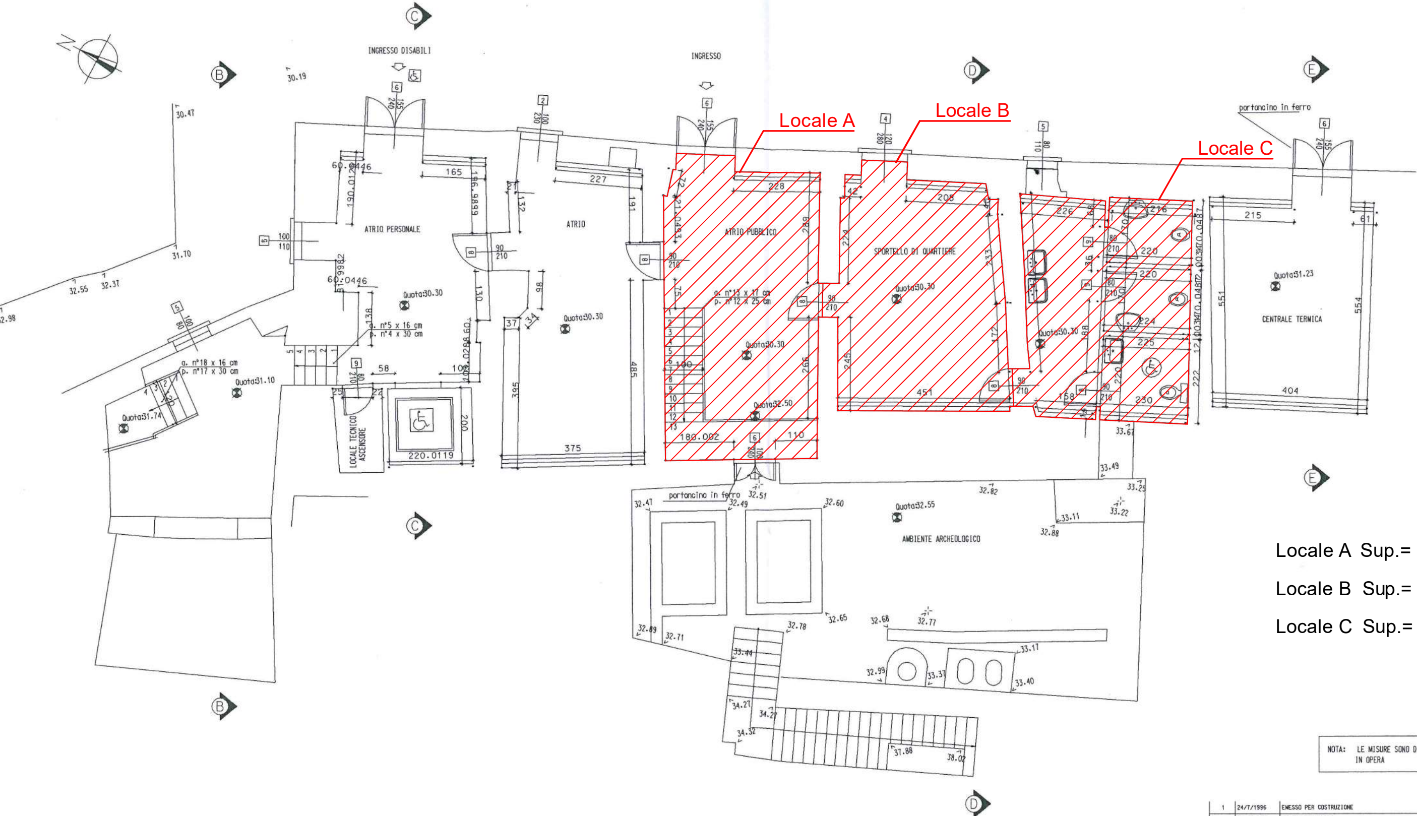
PIANTA QUOTA 30.30
