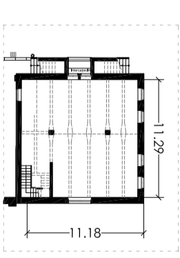
PIANTA PIANO SEMINTERRATO LOCALE TECNICI / CENTRALE TERMORIGORIFERA
