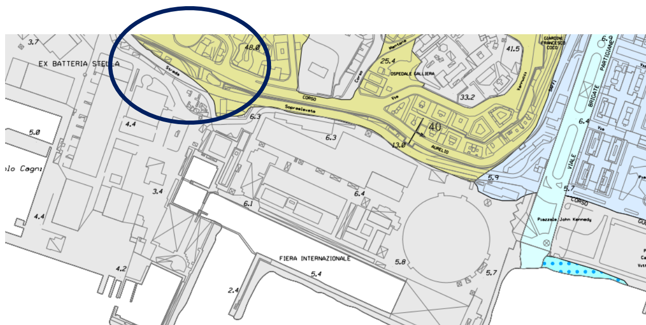
Carta geologica
