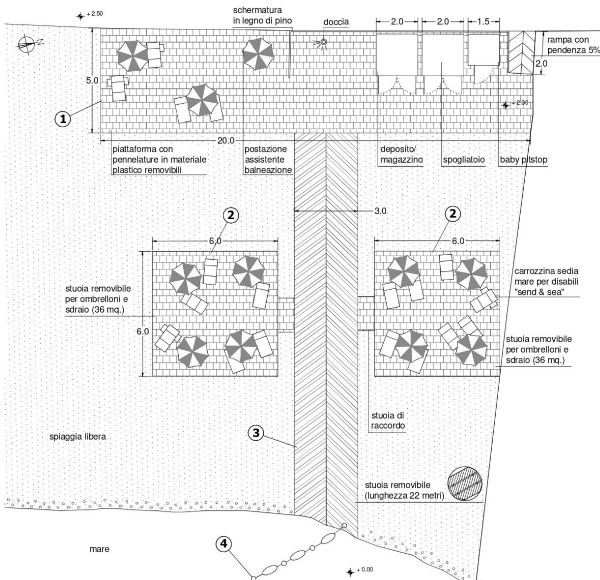
Dettaglio planimetrico di progetto
