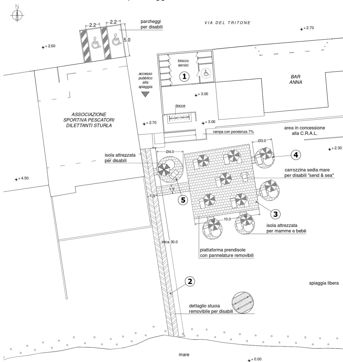
Dettaglio planimetrico di progetto
