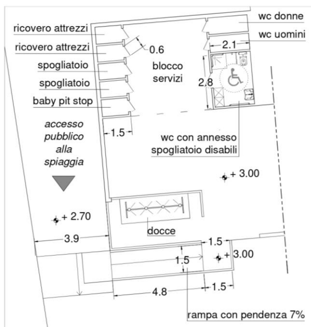
Dettaglio planimetrico del blocco servizi (ipotesi 1) con piatto doccia filo pavimento
