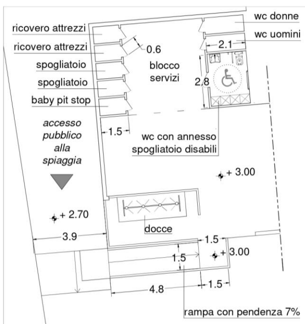
Dettaglio planimetrico del blocco servizi (ipotesi 2) senza piatto doccia filo pavimento
