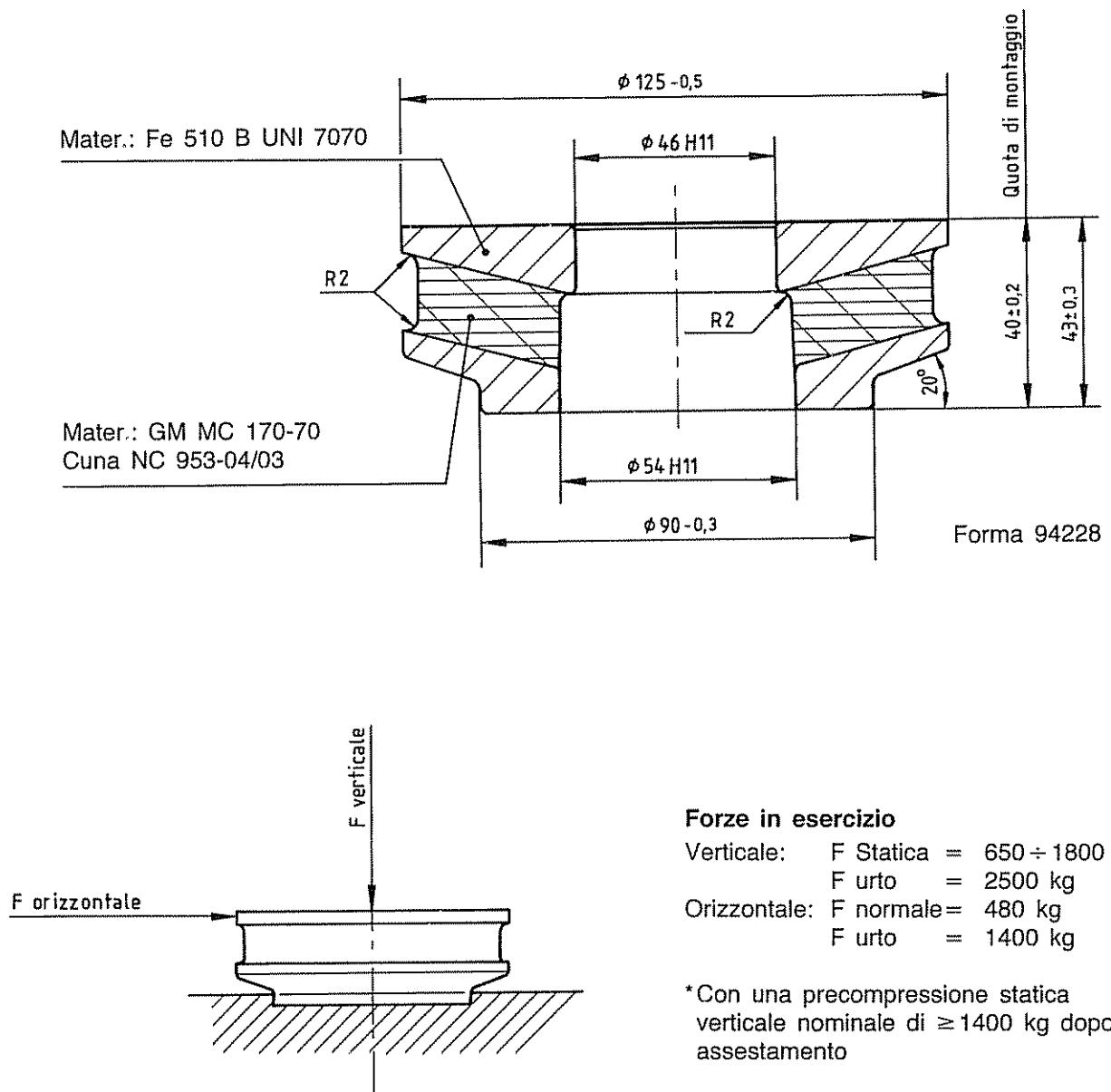
Fig. 11 - Tassello elastico sospensione motore di trazione
