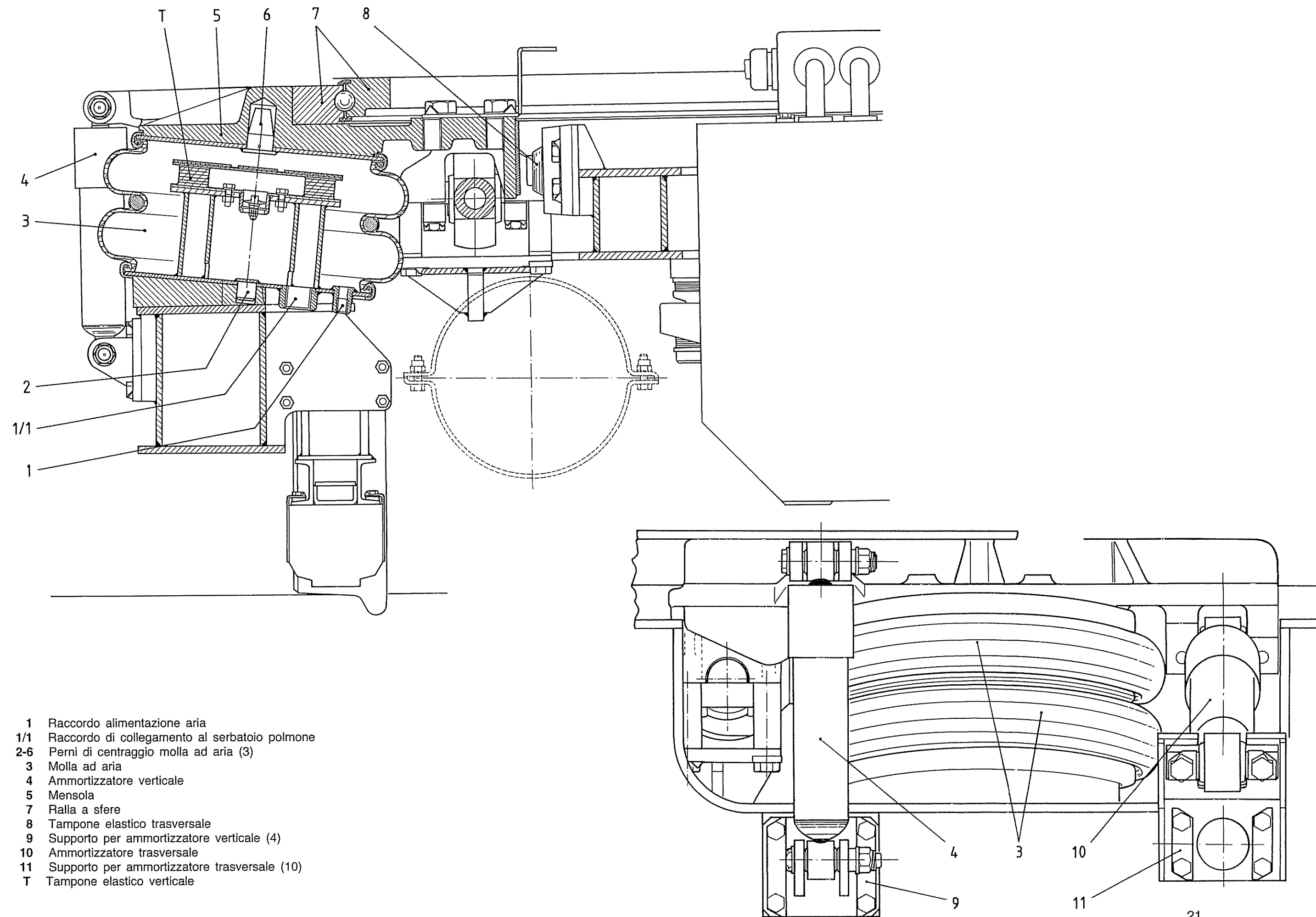
Fig. 6 - Sospensione secondaria
