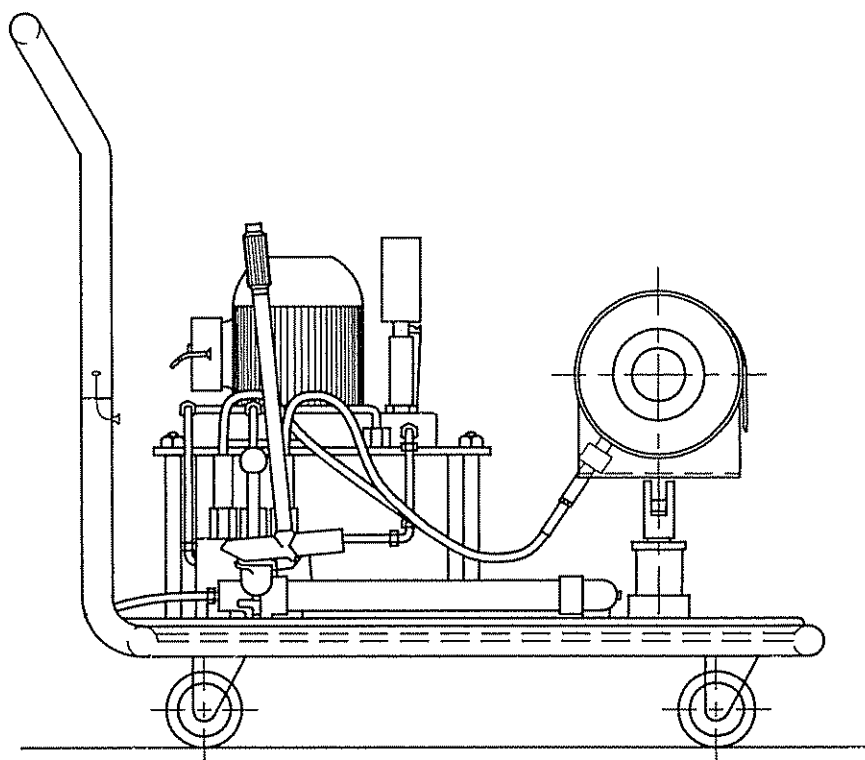
Fig. 9 - Pressa idraulica per montaggio-smontaggio boccole
