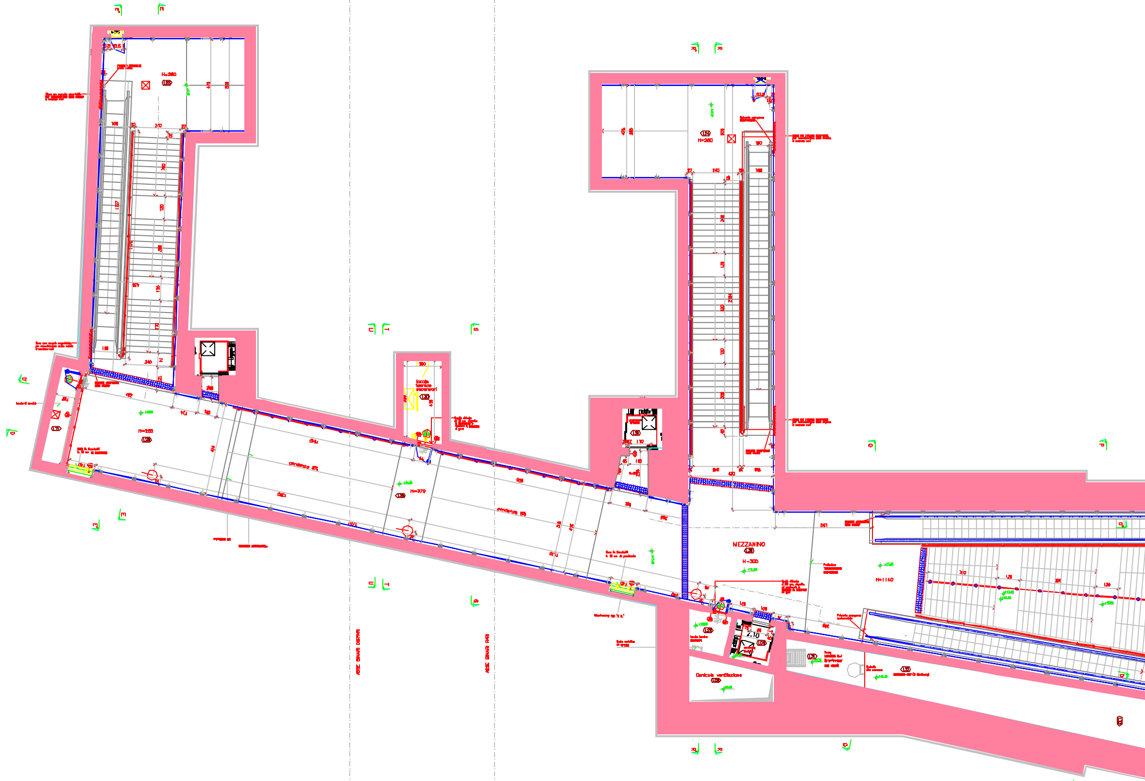
Stazione De Ferrari: Pianta mezzanino e scavalco
