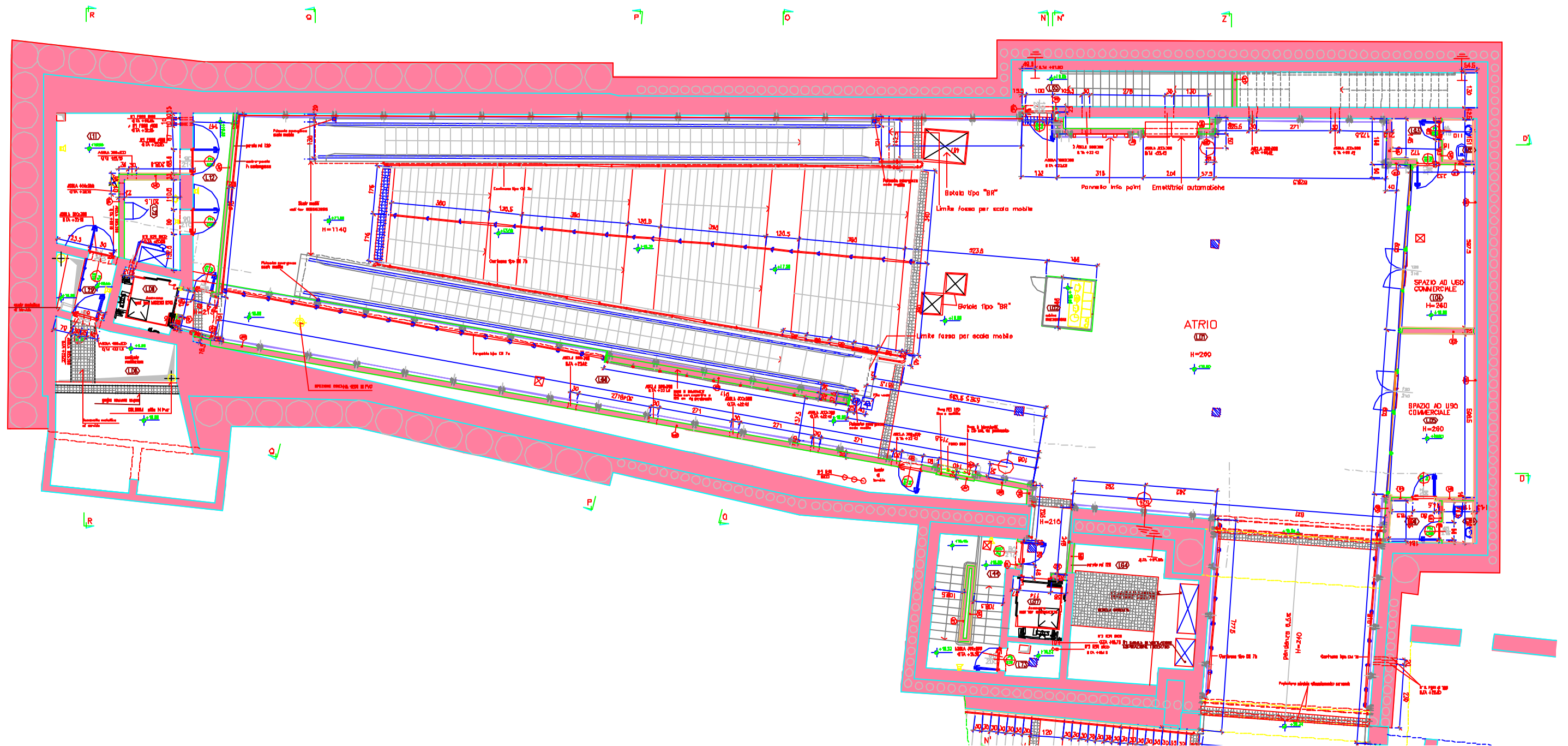
Stazione De Ferrari: atrio e mezzanino
