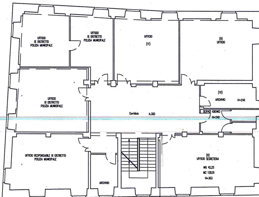
PIANO TERZO
