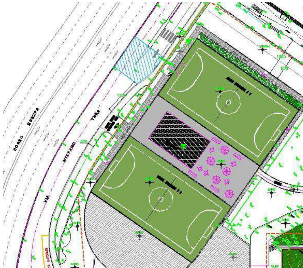
Figura 40. Dettaglio accesso su via Turr
