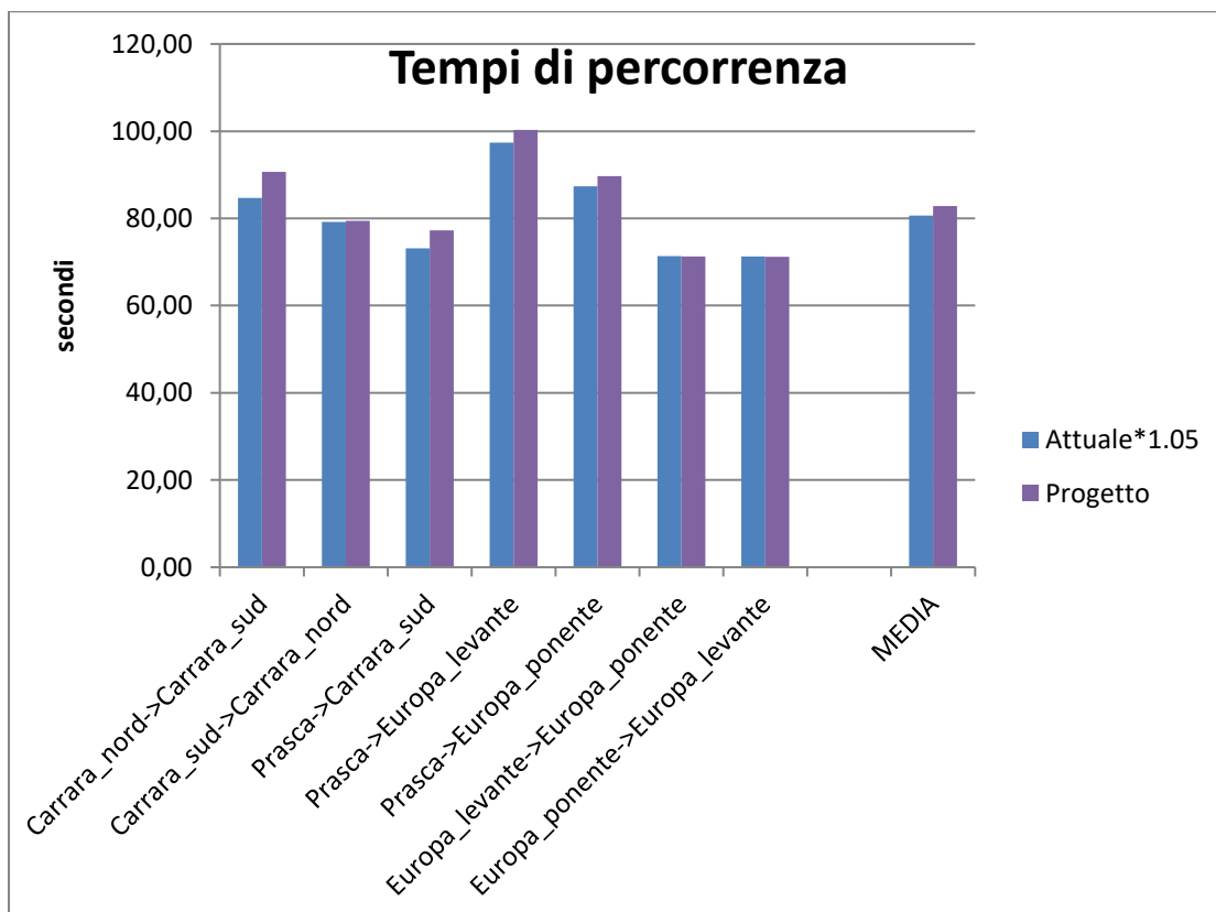
Figura 35. Tempi di percorrenza sui percorsi principali
