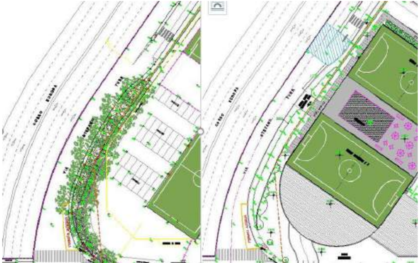
Figura 41. Sistemazione via Turr: stato di fatto (a sinistra) e progetto (a destra)
