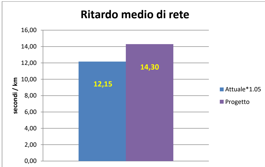
Figura 32. Ritardo medio di rete nei due scenari
