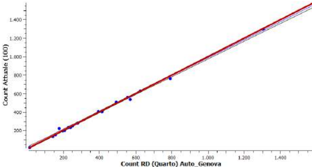
Figura 17. Regressione lineare dei valori dei volumi di traffico misurati e stimati sulle sezioni
