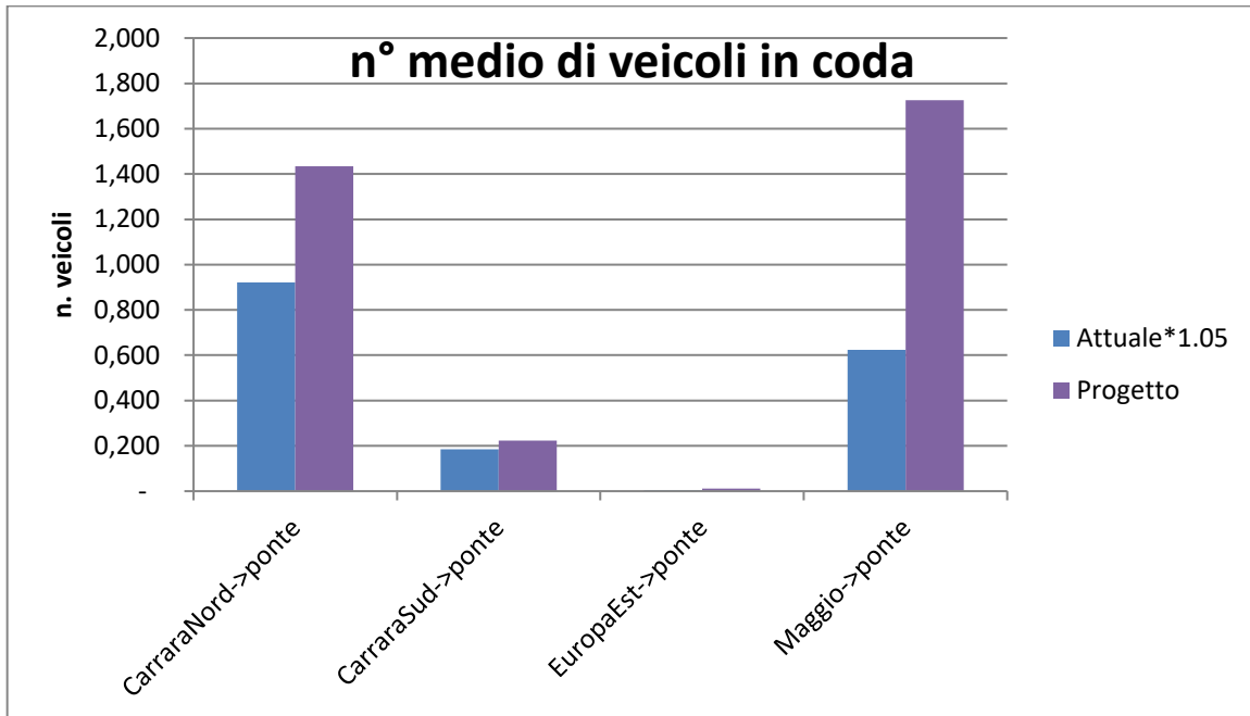
Figura 33. code medie sugli attestamenti critici
