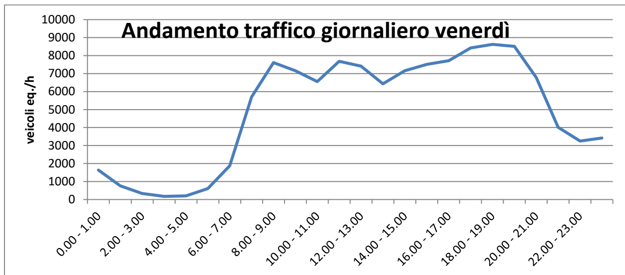
Figura 9. andamento traffico totale nella giornata di venerdì
