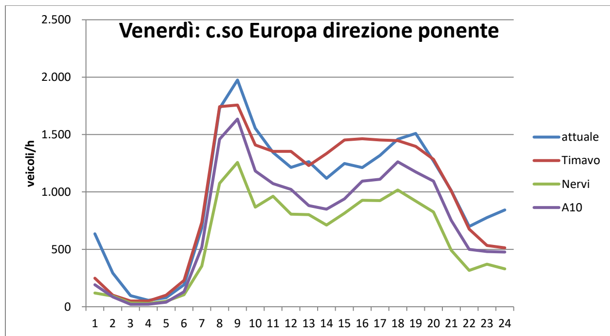
Figura 13. Andamenti sulle sezioni direzione ponente
