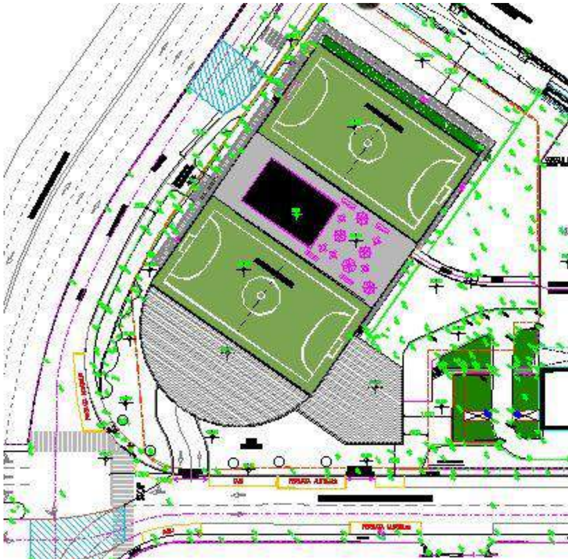
Figura 3. Planimetria del progetto
