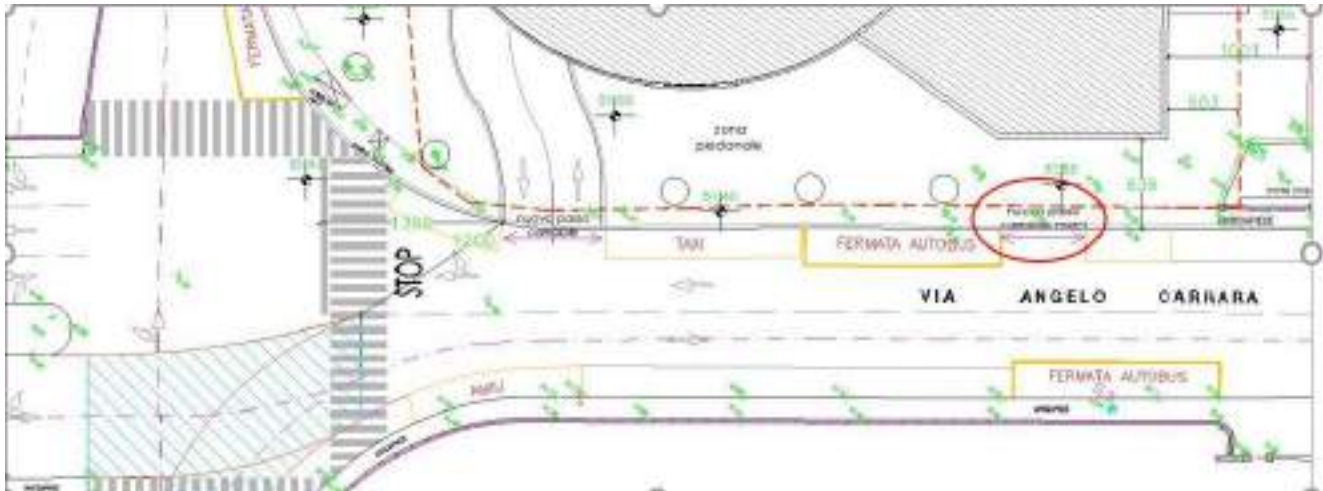
Figura 38. Dettaglio accesso via Carrara con distanze dall’intersezione
