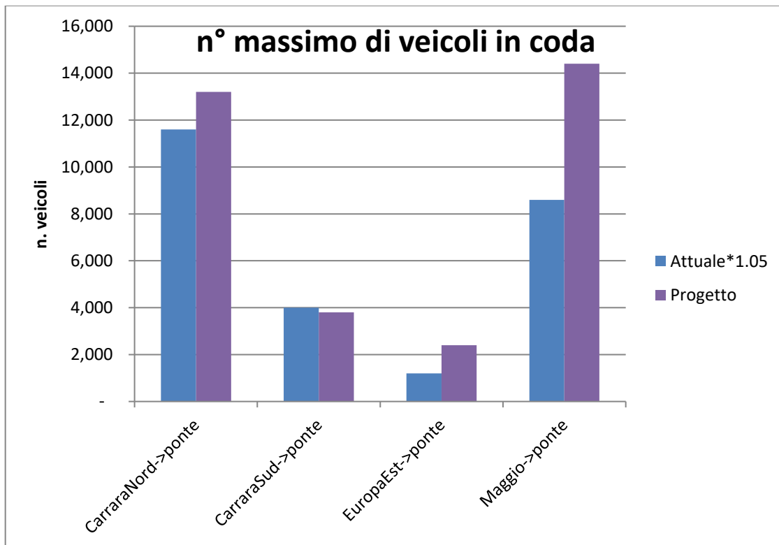
Figura 34. Code massime sugli attestamenti critici
