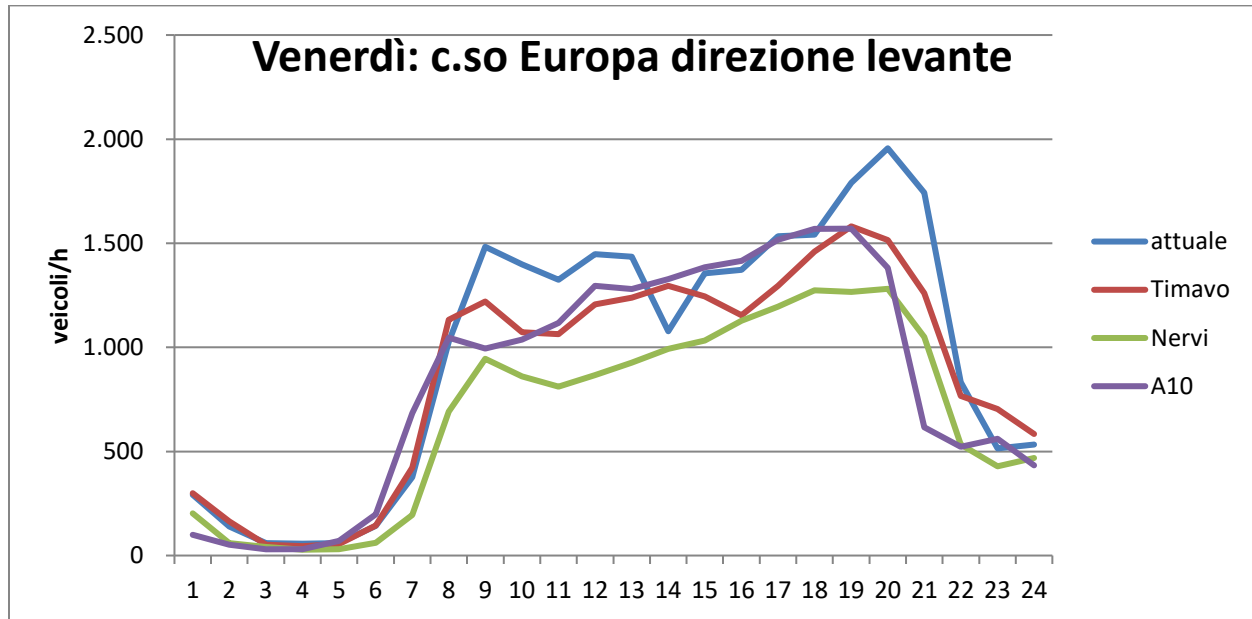
Figura 12. Andamenti sulle sezioni direzione levante
