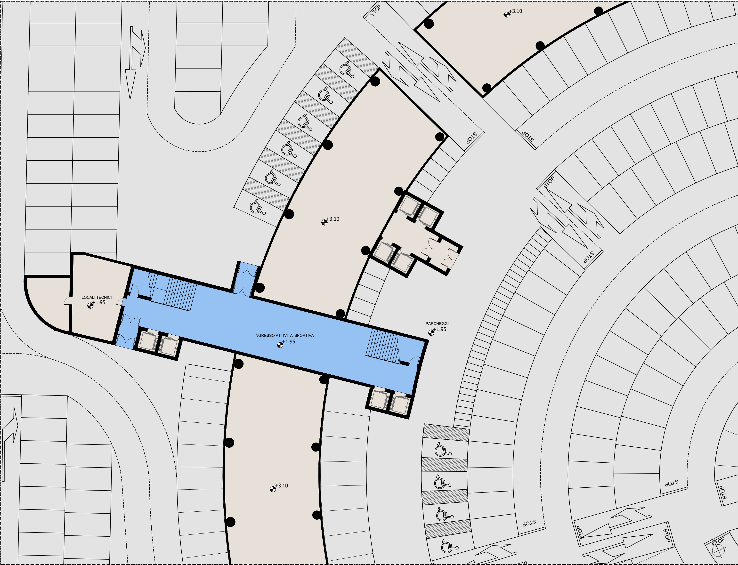
STRALCIO PIANTE PIANO INTERRATO QUOTA + 1.95
