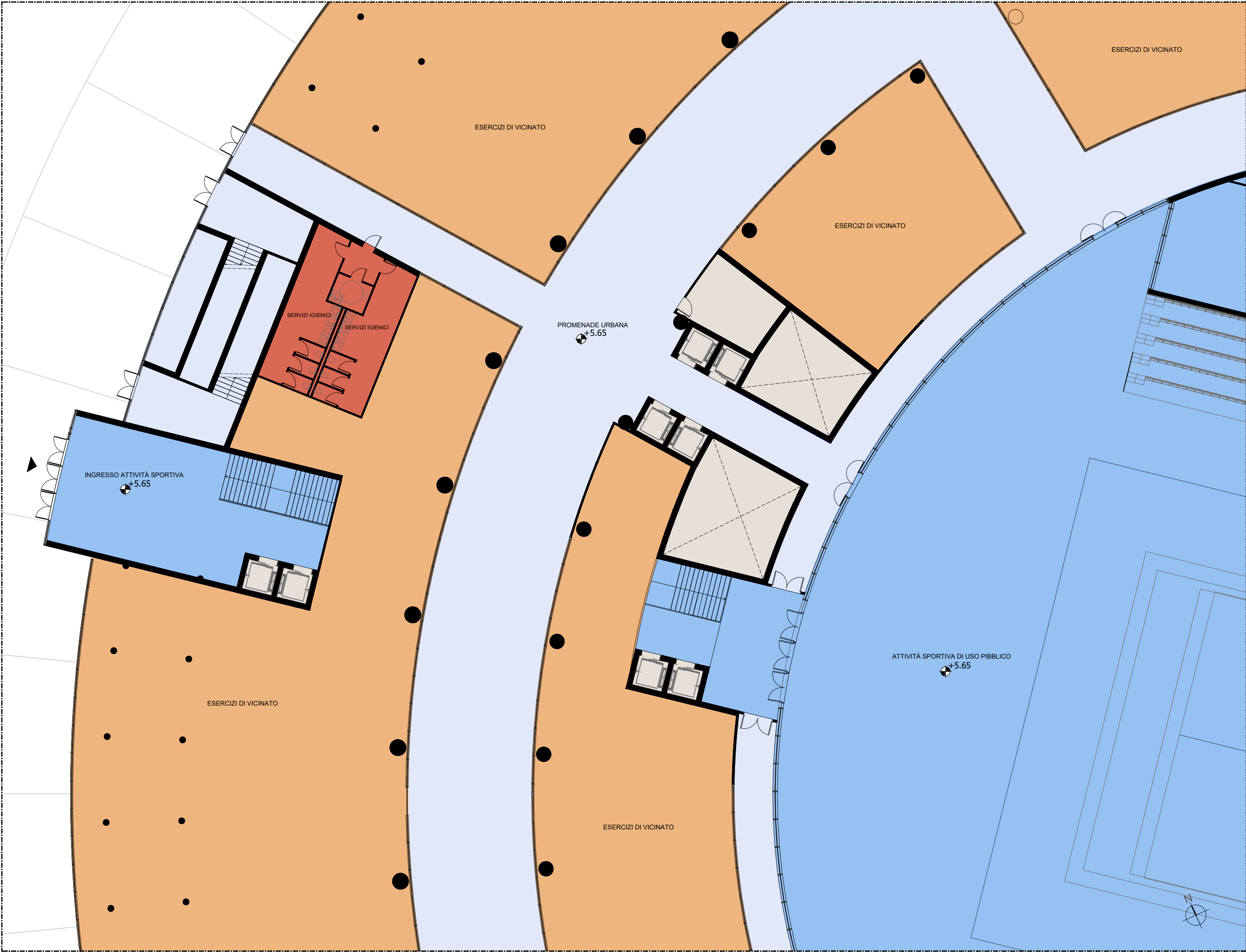
STRALCIO PIANTE PIANO TERRA QUOTA + 5.65
