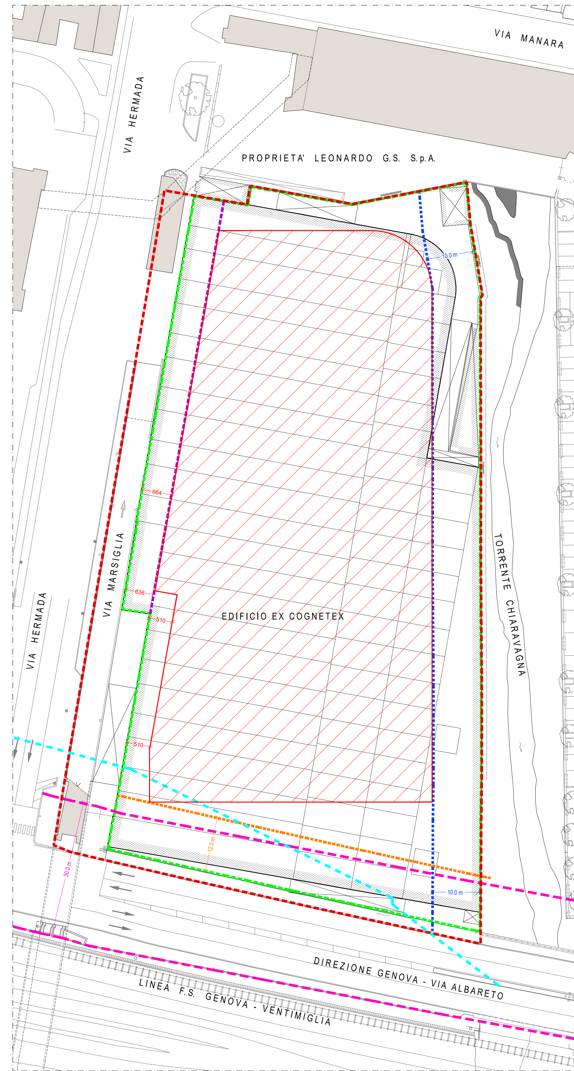
SOVRAPPOSIZIONE IMPRONTA NUOVA EDIFICAZIONE SU RILIEVO DELLO STATO DI FATTO
