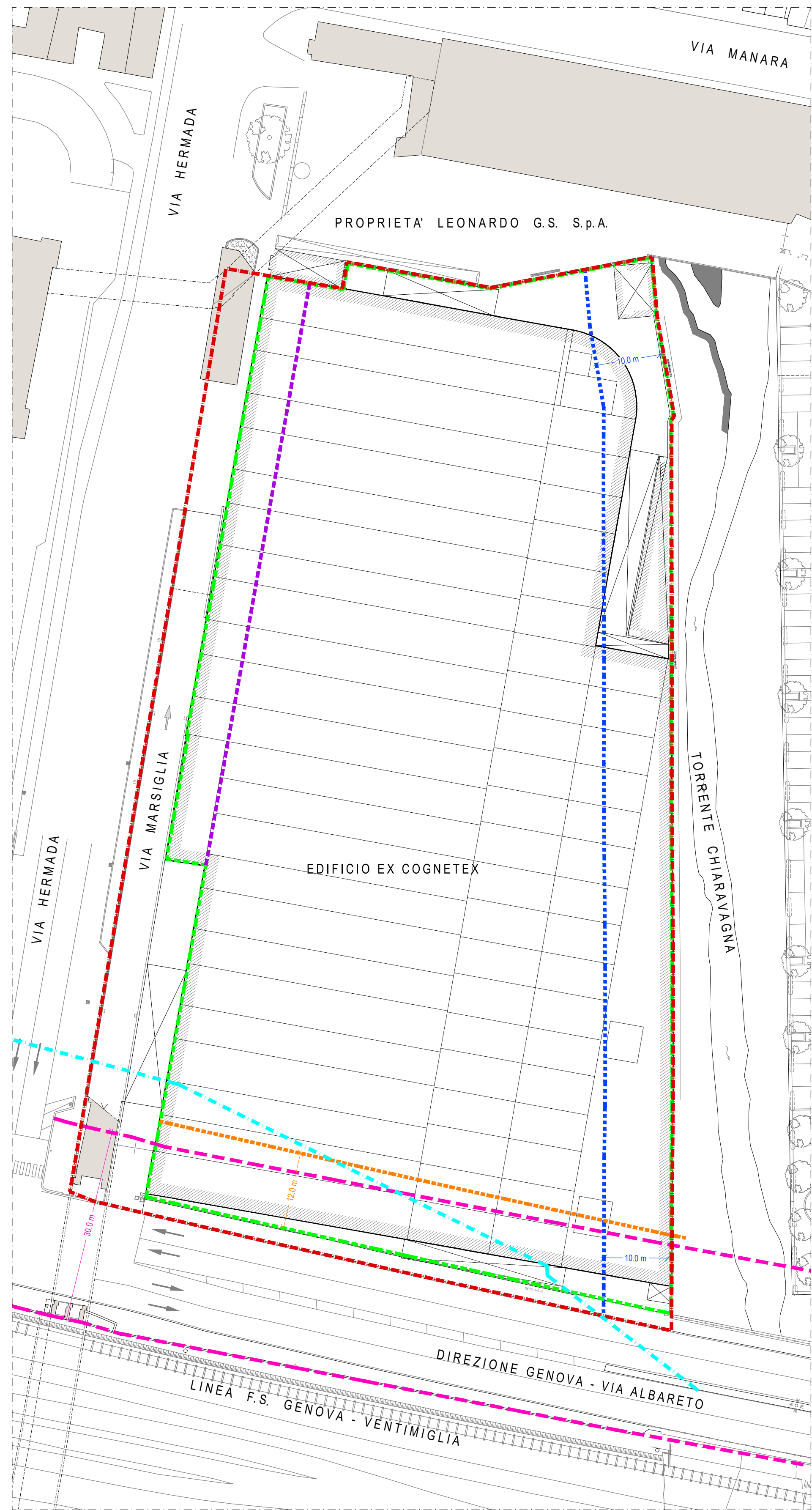
RILIEVO DELLO STATO DI FATTO
