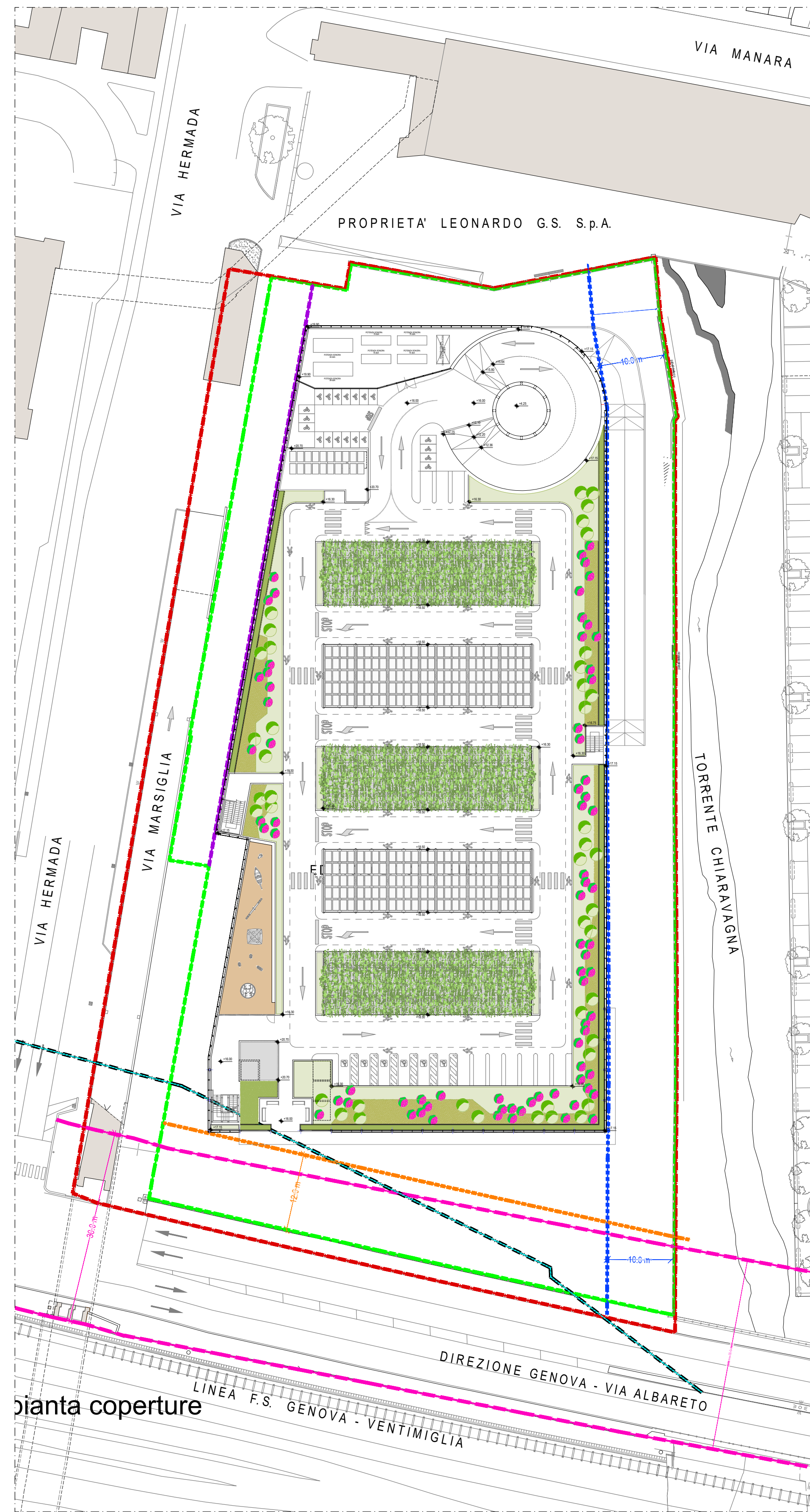
PLANIMETRIA GENERALE DELLE COPERTURE
