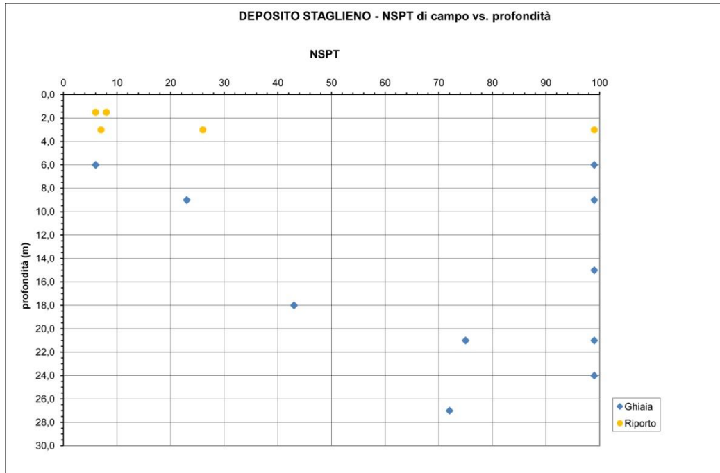
Figura 12. Deposito Staglieno: grafico NSPT - Profondità
