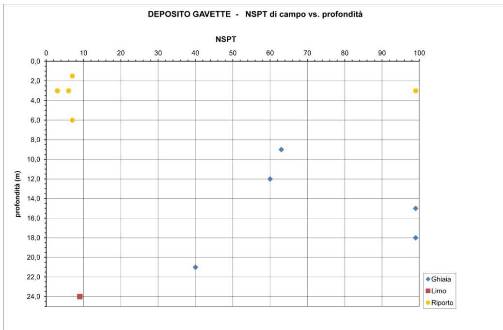
Figura 13. Deposito Gavette: grafico NSPT - Profondità
