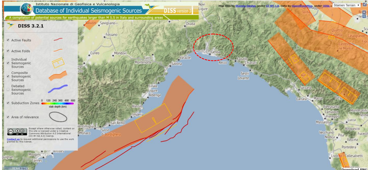
Figura 19. Sorgenti sismogenetiche contenute nella nuova versione del “Database of Potential Sources for Earthquakes larger than M 5.5 in Italy” – Immagine focalizzata sull’ambito ligure. In rosso l’area di studio. ( http://diss.rm.ingv.it/diss/ ).
