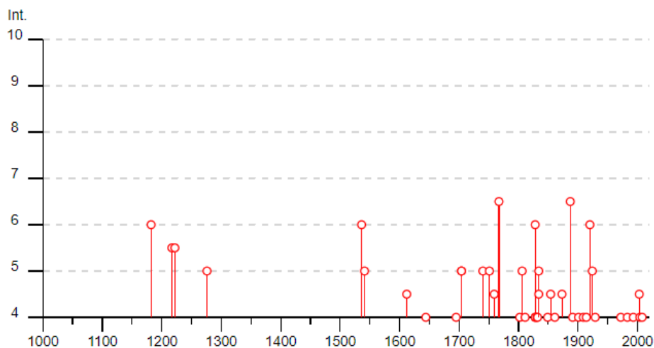
Figura 18. Sismicità storica del Comune di Genova [44.419, 8.898] 131 eventi nel periodo 1000-2020 - intensità massima registrata 6-7.
