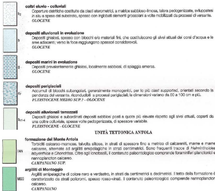
Figura 9. Stralcio del Foglio Genova 213, progetto CARG, della Carta Geologica d'Italia.
