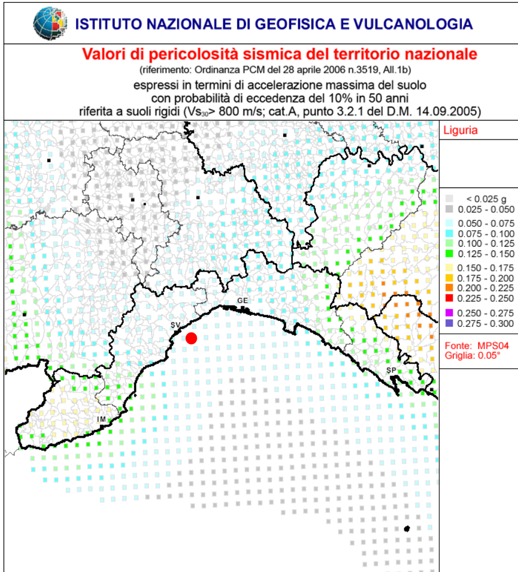
Figura 17. Mappa di pericolosità sismica espressa in termini di accelerazione massima del suolo ( a_{max} ) con probabilità di eccedenza del 10% in 50 anni riferita a suoli molto rigidi ( V_{s30} > 800\text{ m/s} ) – da INGV. In rosso l'area di studio.
