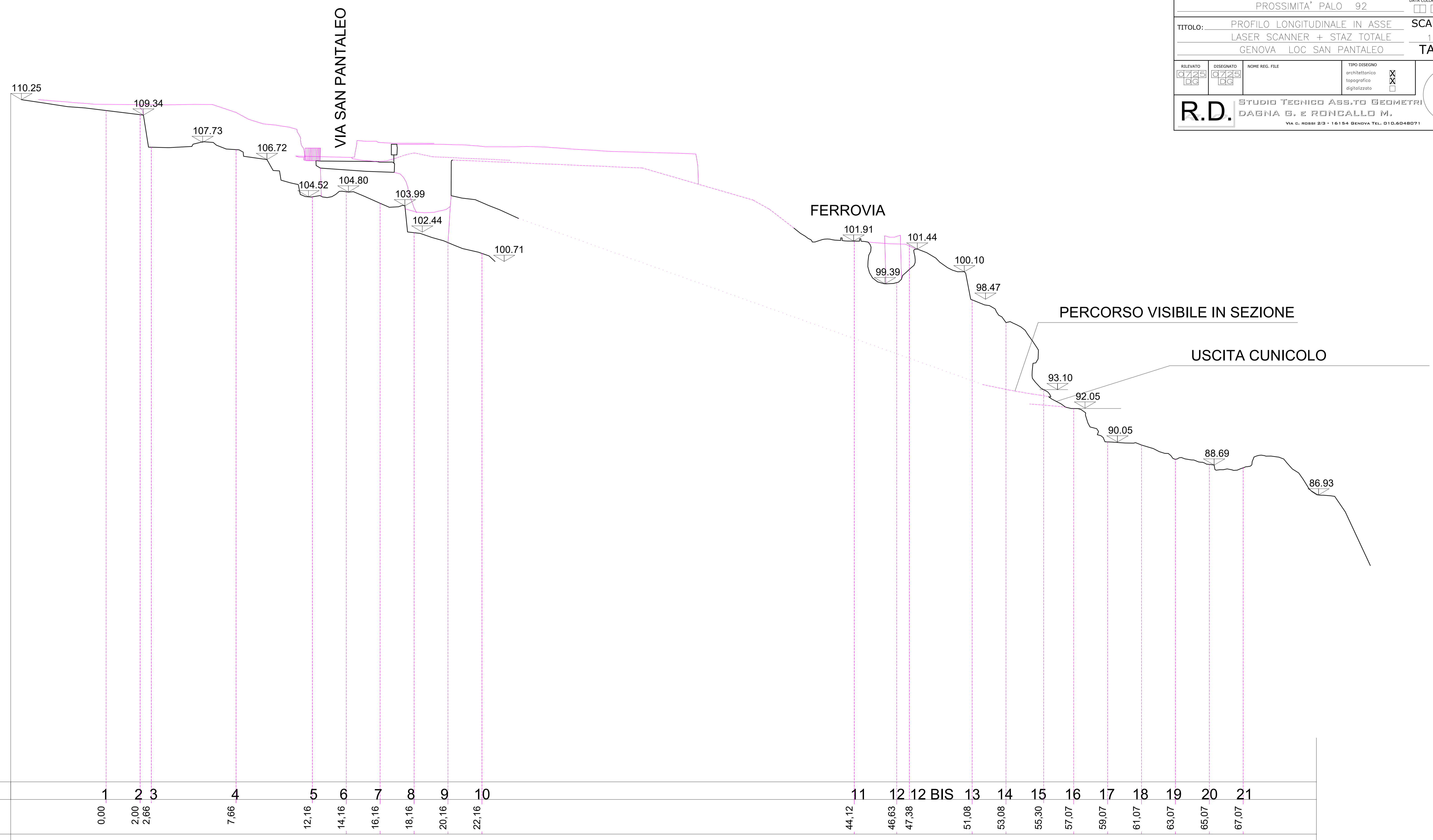
PROFILO LONGITUDINALE
