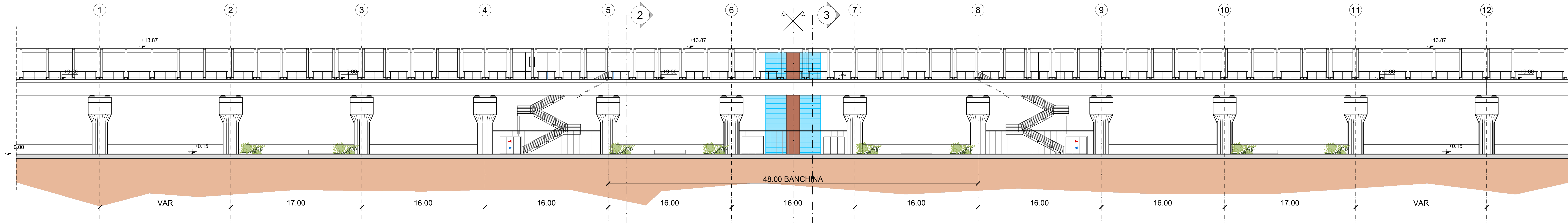
PROSPETTO LONGITUDINALE
