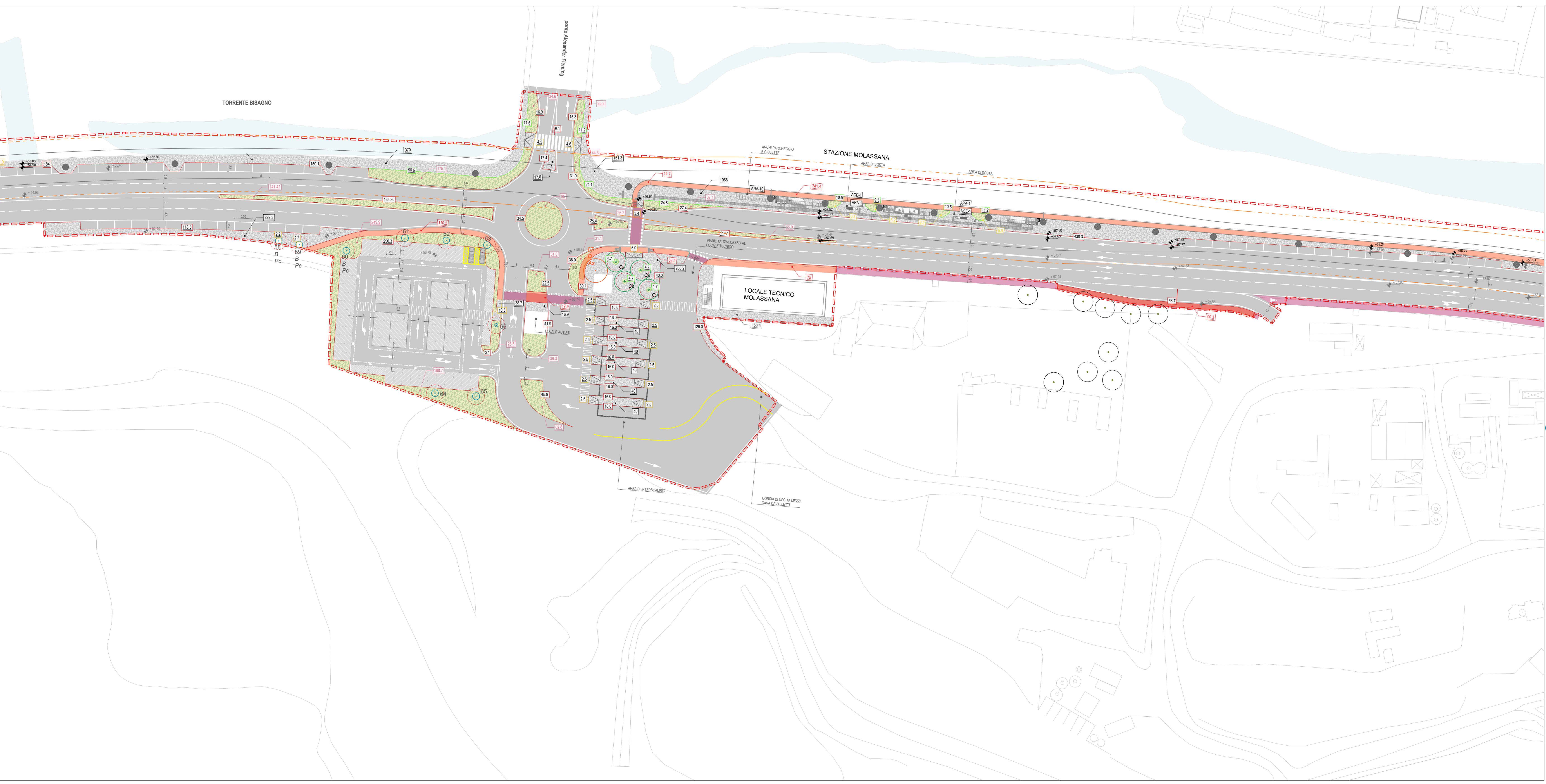
01 PLANIMETRIA GENERALE 1:500
