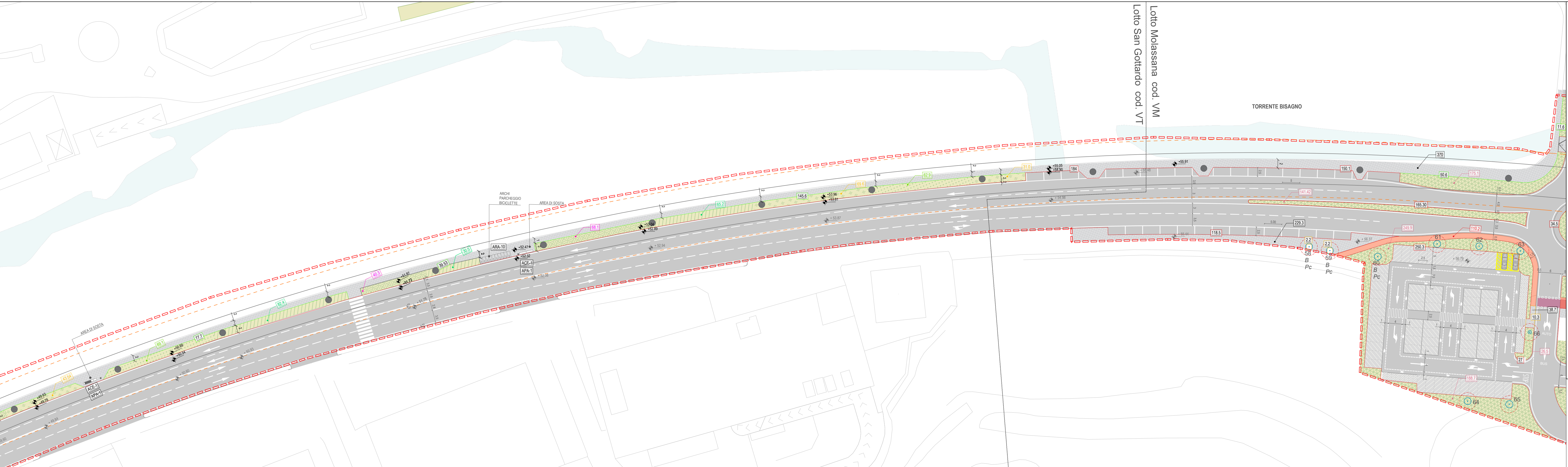
01 PLANIMETRIA GENERALE 1:500
