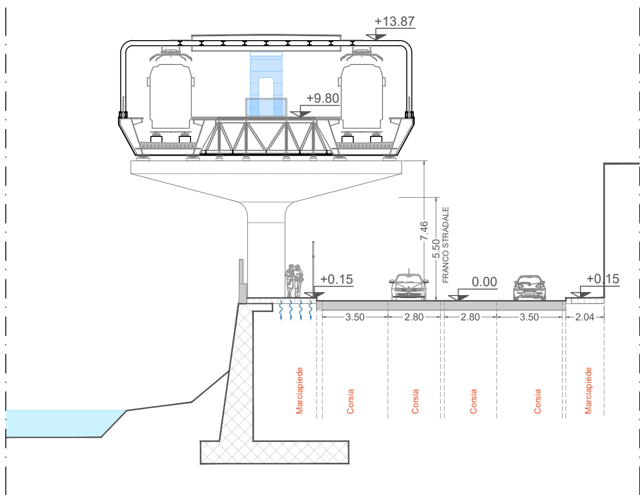
S02 SEZIONE TRASVERSALE TIPOLOGICA AA' Scala 1:200 STATO DI PROGETTO
