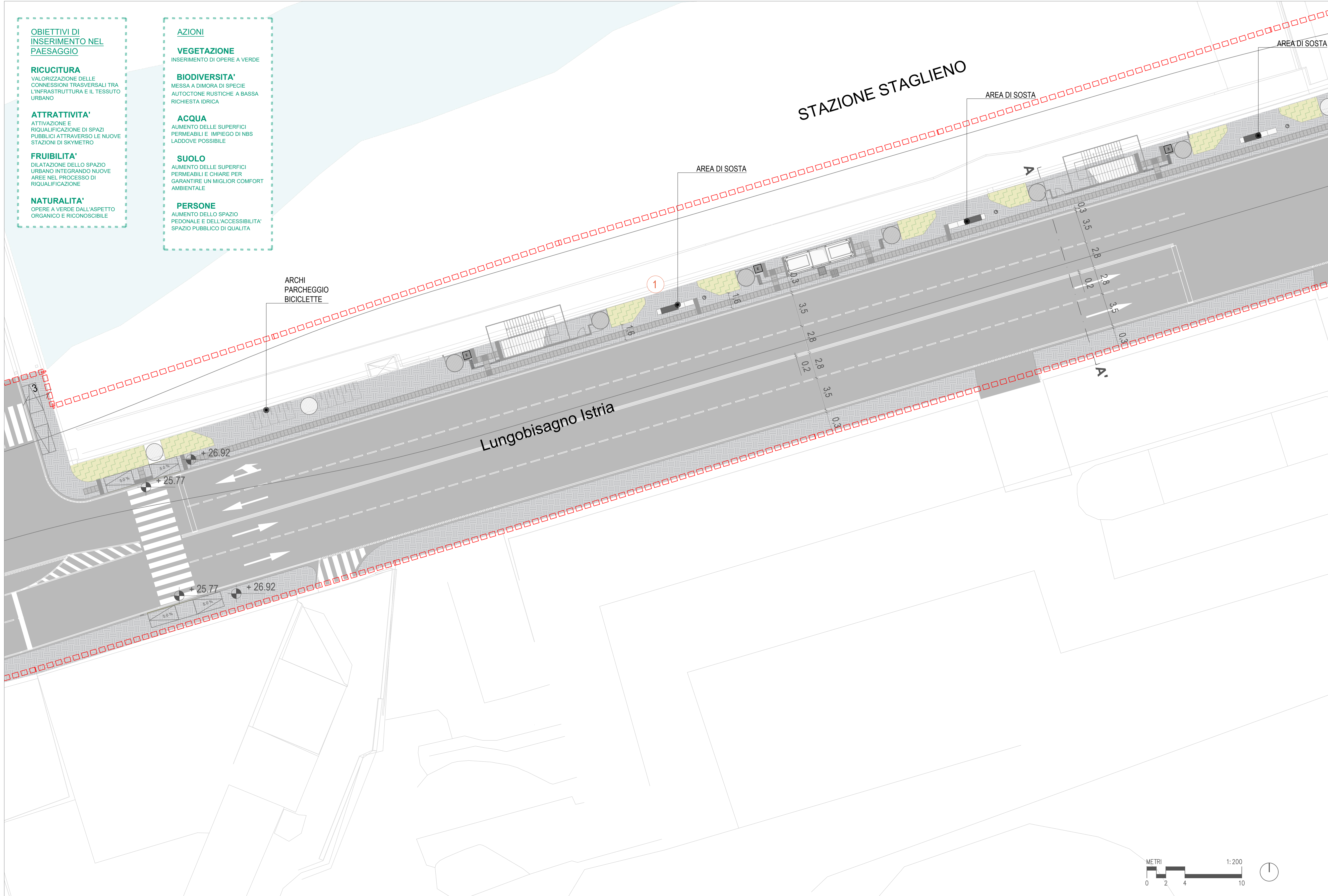
P02 PLANIMETRIA Scala 1:200 STATO DI PROGETTO
