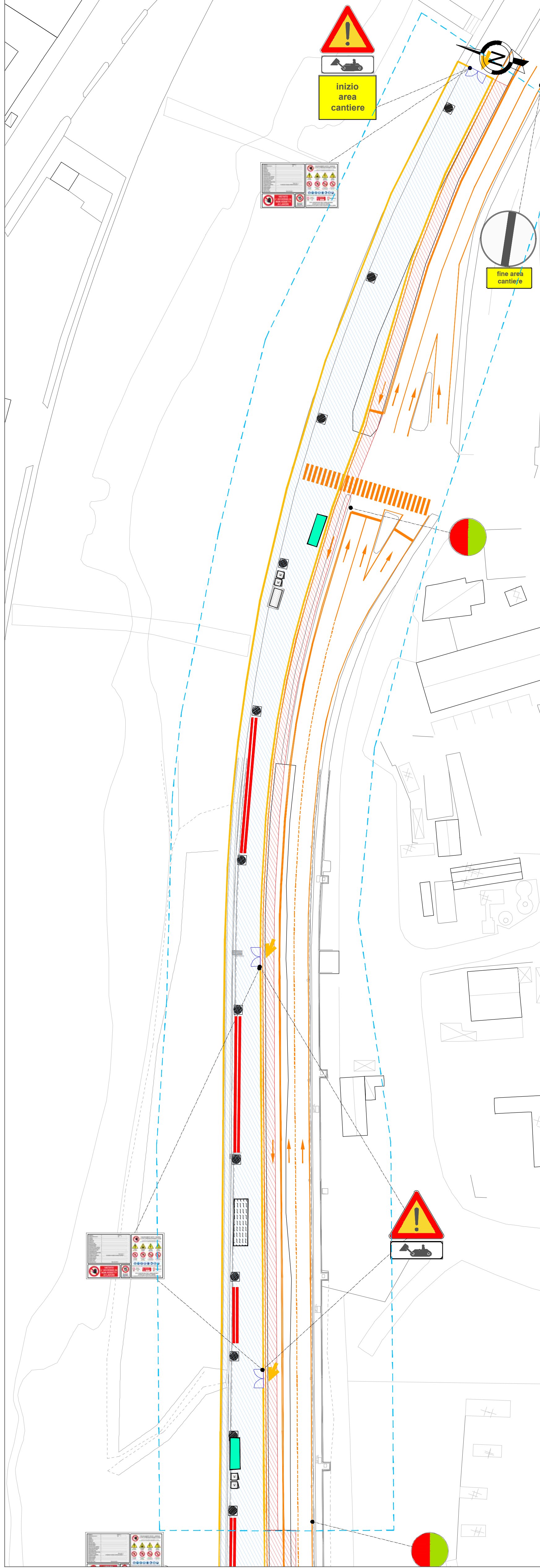
CANT A0 - FASE 3 - scala 1:500 - Ampliamento per porzioni del cantiere, con conseguente diminuzione della sezione stradale e istituzione di senso unico alternato in notturna. - Costruzione e posa degli impalcati, con posa notturna dello stesso per tratti, attraverso la chiusura di una porzione di carreggiata e il posizionamento di movieri per il controllo del traffico a senso alternato. - Realizzazione delle travature di collegamento e della soletta degli impalcati - Realizzazione OO.CC. stazione VIABILITA' - Chiusura una corsia in direzione sud su via Gelasio Adamoli VIABILITA' ALTERNATIVA - Via Molassana
