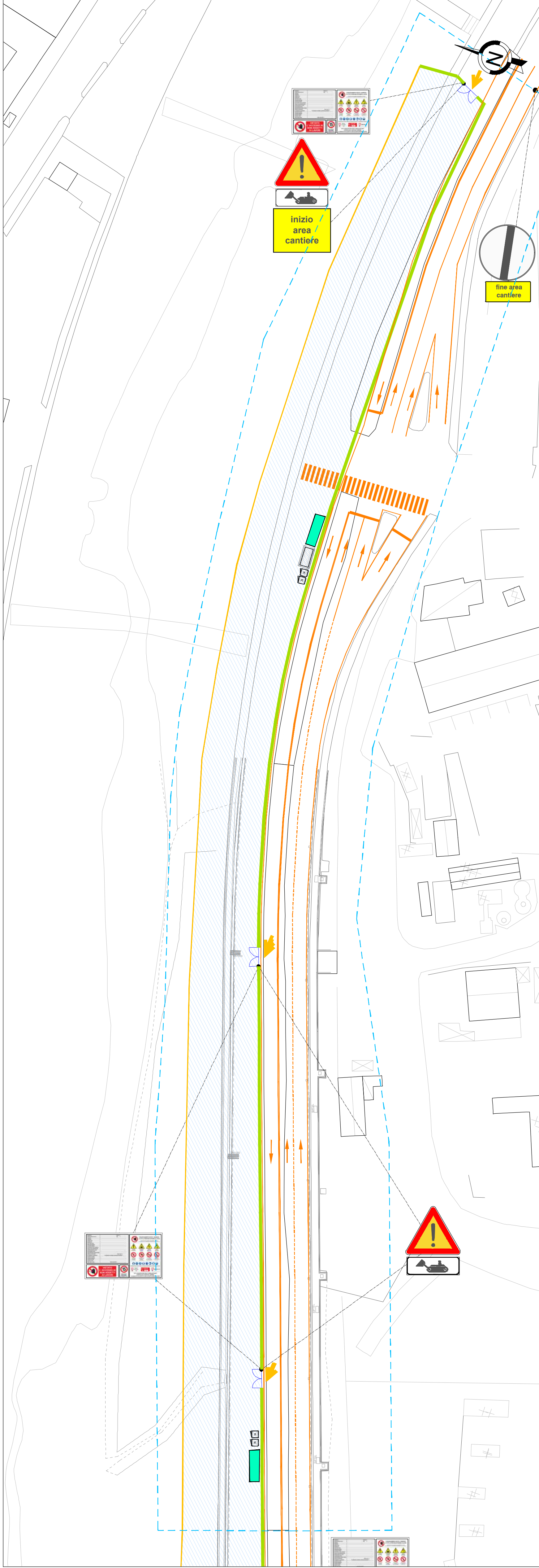
CANT A0 - FASE 2 - scala 1:500 - ampliamento cantiere all'interno dell'alveo - Demolizioni porzioni di argine - Realizzazioni pile e pulvino - Realizzazioni sistemazioni urbane lato nord VIABILITA' - Chiusura una corsia in direzione sud su via Gelasio Adamoli VIABILITA' ALTERNATIVA - Via Molassana
