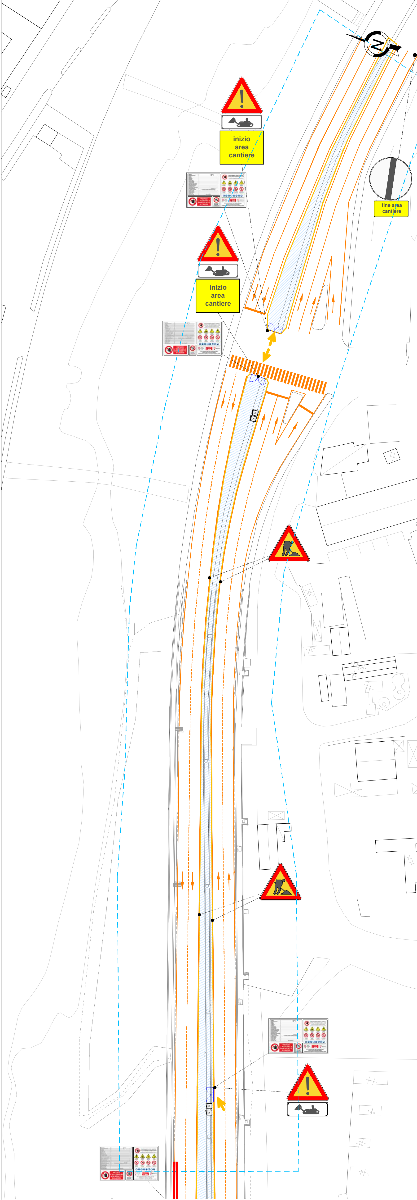
CANT A0 - FASE 0 - scala 1:500 - Realizzazione layout di cantiere - Demolizione cordolo spartitraffico centrale - Asfaltatura area interessata dal cordolo - Realizzazione segnaletica orizzontale provvisoria
