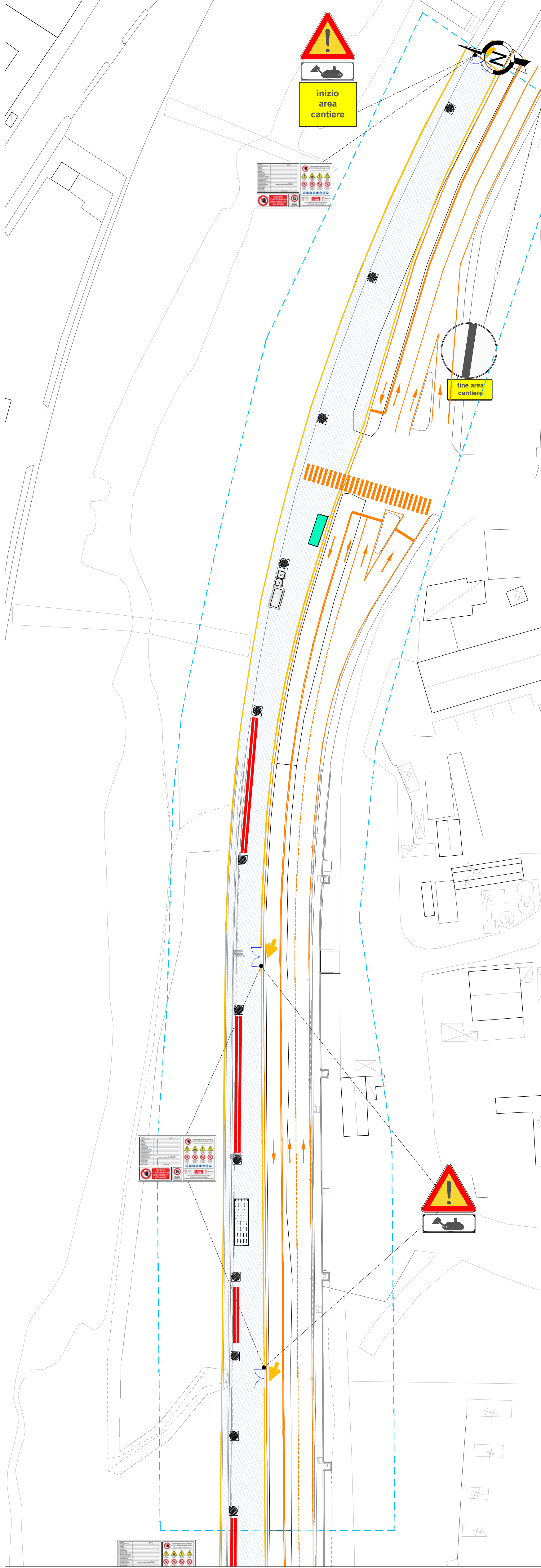
CANT A0 - FASE 4 - scala 1:500 - Realizzazione armamento - Realizzazione impianti - realizzazione finiture - Completamento stazione VIABILITA' - Chiusura una corsia in direzione sud su via Gelasio Adamoli VIABILITA' ALTERNATIVA - Via Molassana
