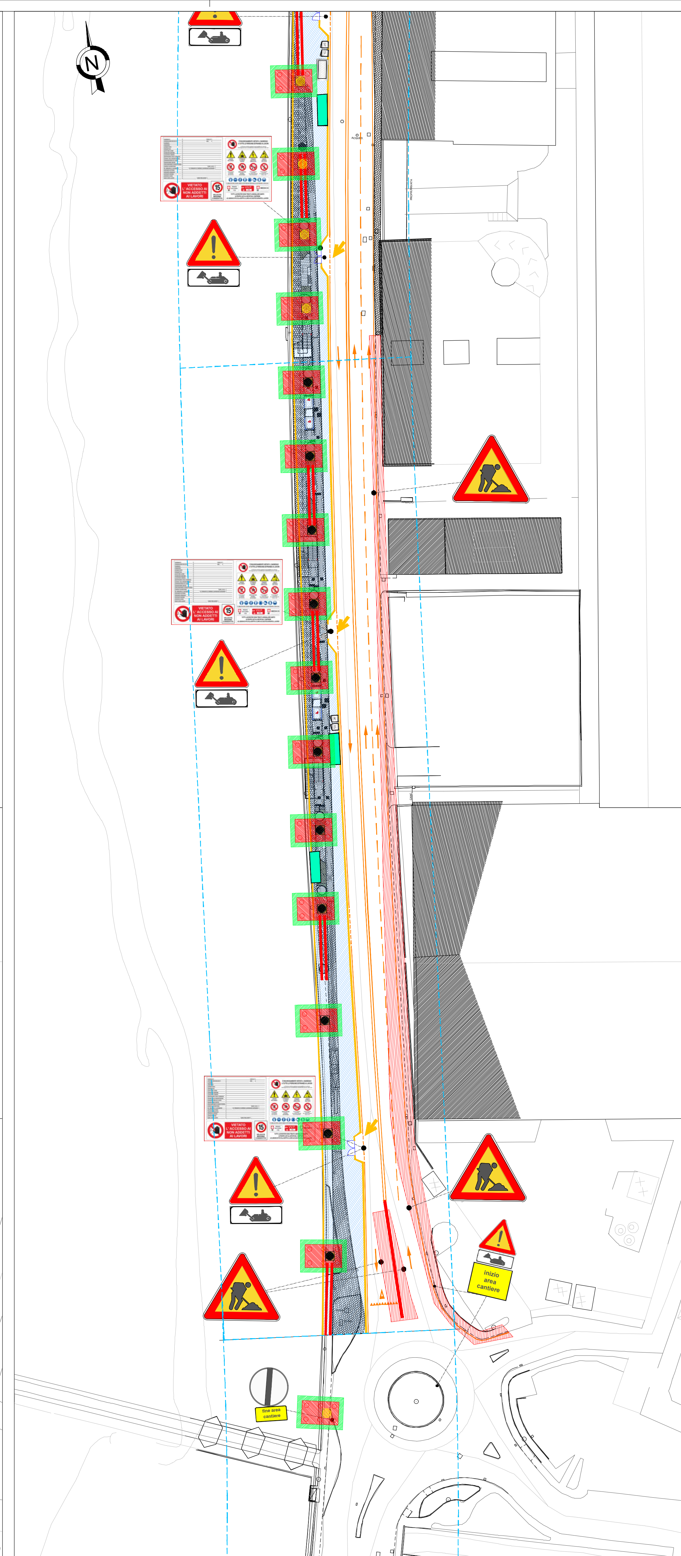
CANT B4 - FASE 4-1 - scala 1:500
