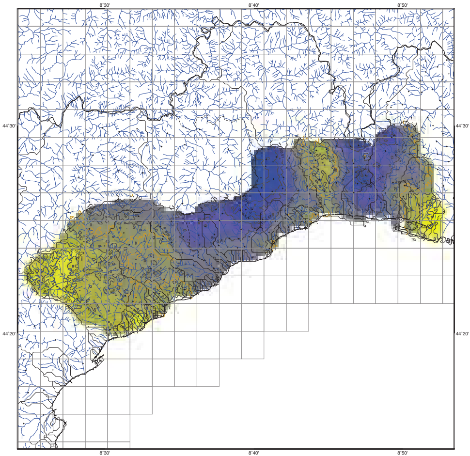
CARTA GEOLITOGICA Scala 1:33333 Riclassificata da Modello Strutturale
