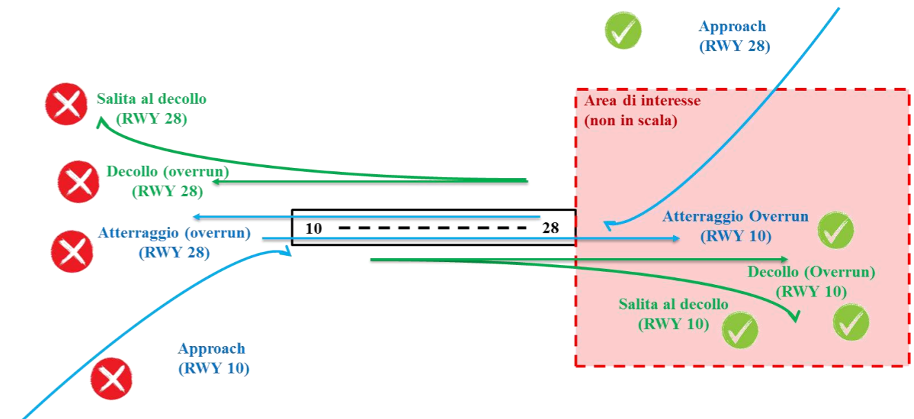
Figura 5.4. Fasi del volo considerate
