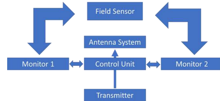
Figura 4.18 Schema esemplificativo del sistema
