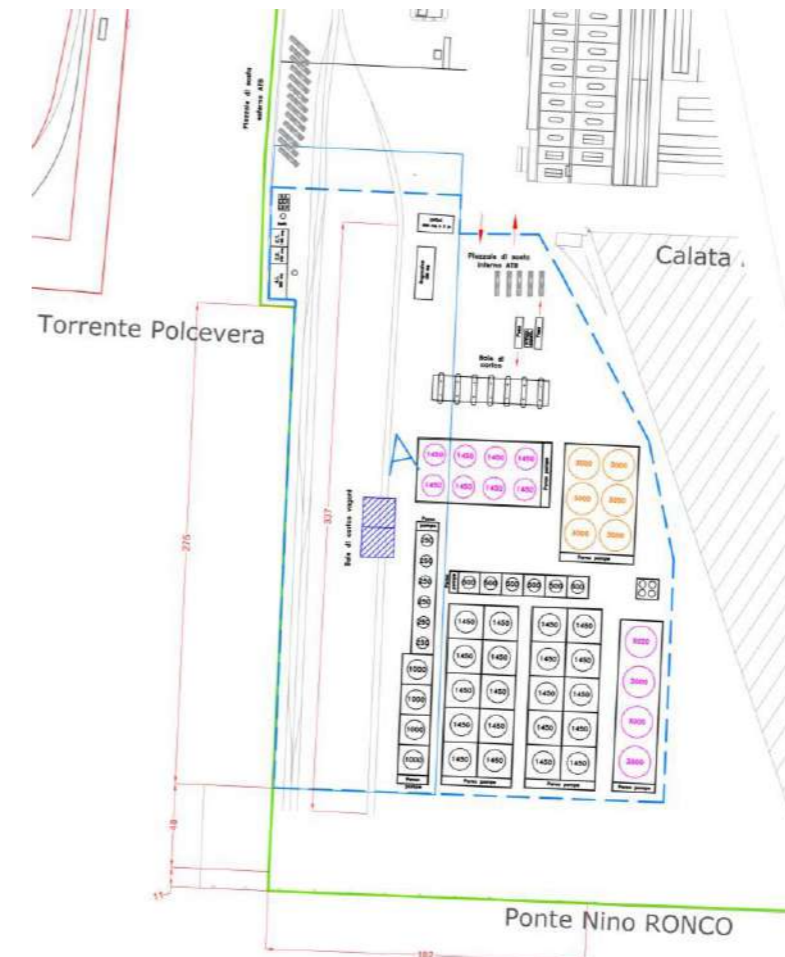
Figura 3.1 Esempificazione di un possibile layout nuova area di deposito Terminal Messina [redacted]
