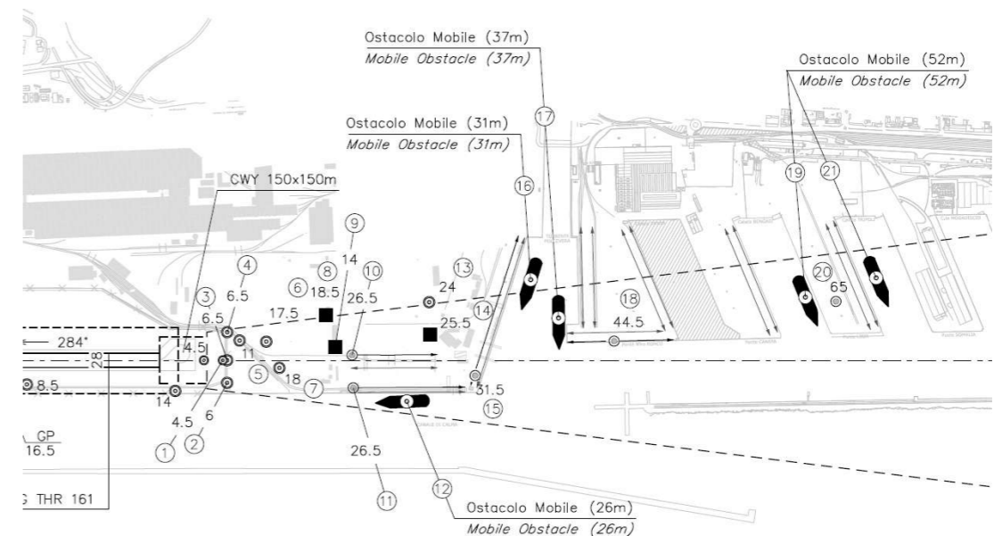
Figura 4.15 Estratto planimetria TOFPA – AIP Italia
