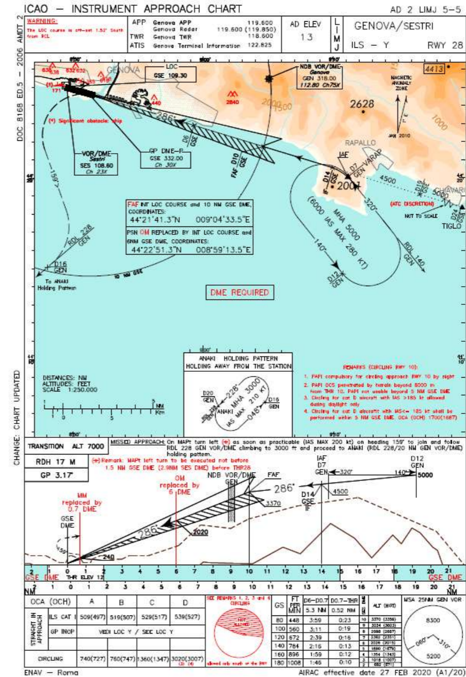
Figura 4.19 ILS-Y RWY28 – AIP ITALIA A1/20
