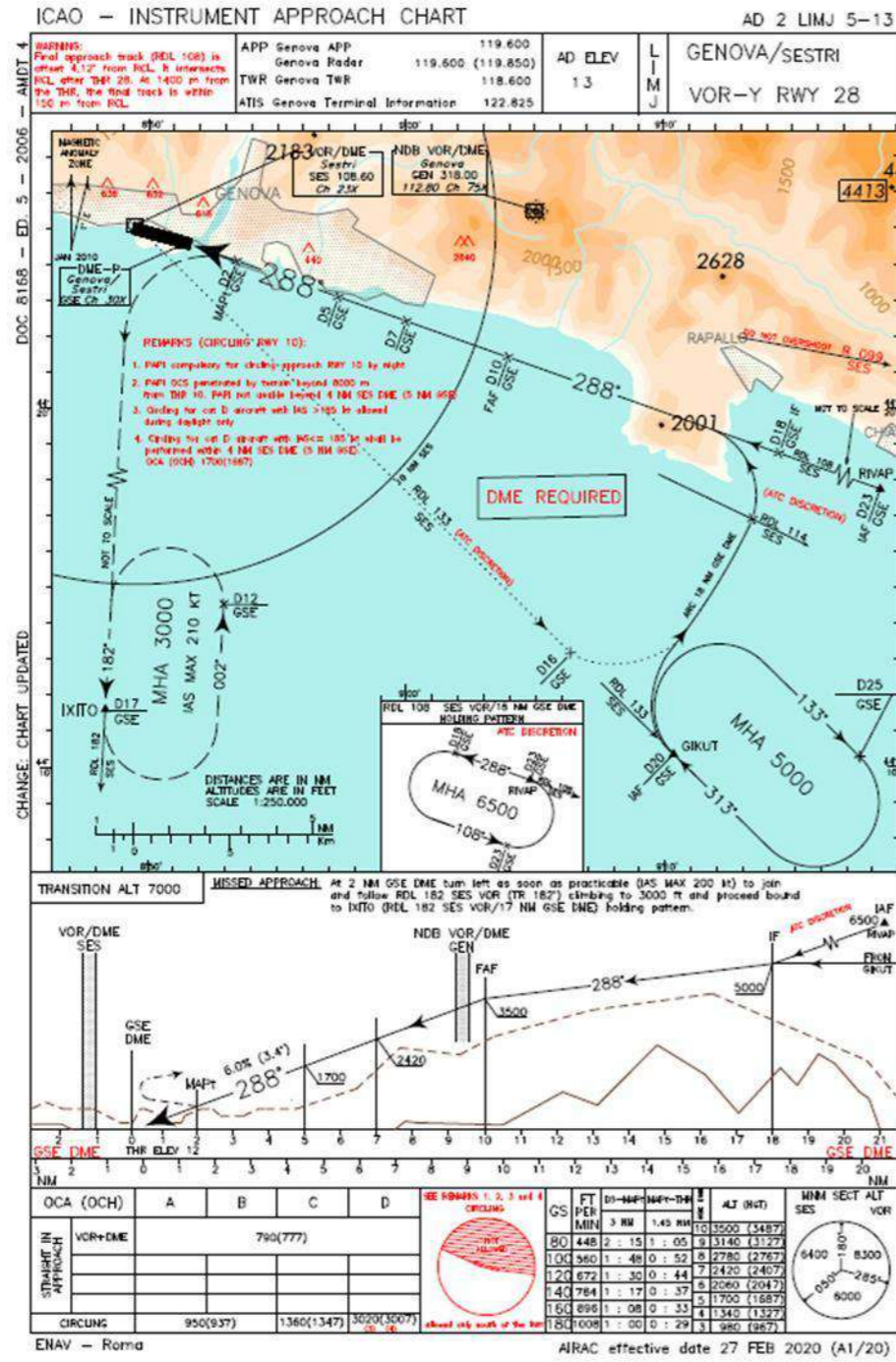
Figura 4.21 VOR-Y RWY28 – AIP ITALIA A1/20
