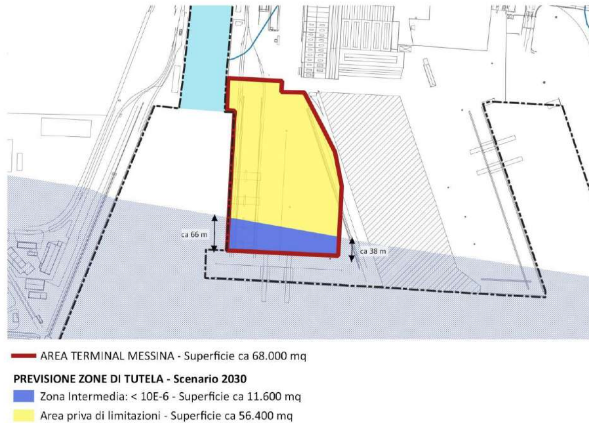
Figura 6.2 Individuazione aree di iso-rischio – Area Terminal Messina
