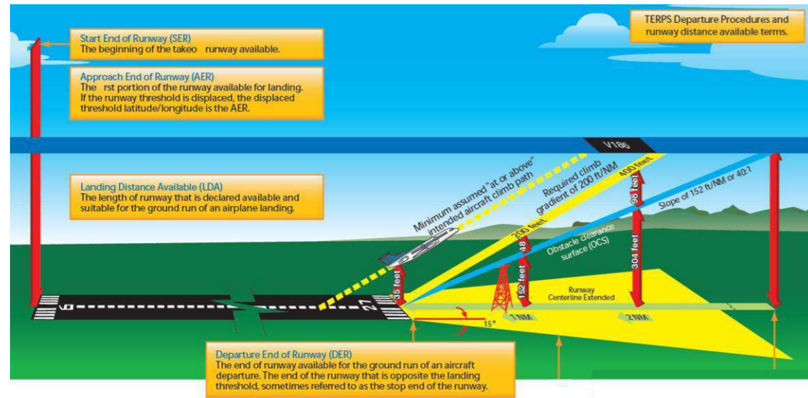
Figura 4.16 Illustrazione schematica della fase iniziale della salita al decollo
