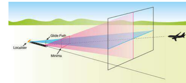
Figura 4.17 Illustrazione schematica di un sistema ILS
