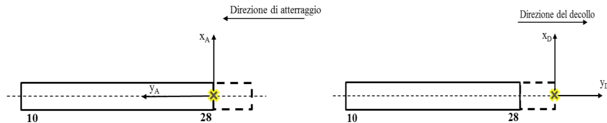
Figura 5.6. Sistema di coordinate per le operazioni di atterraggio e decollo
