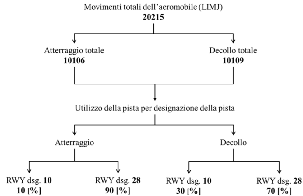
Figura 5.5. Movimenti annuali Aeroporto di Genova suddivisi per fasi di volo (input - anno 2019)
