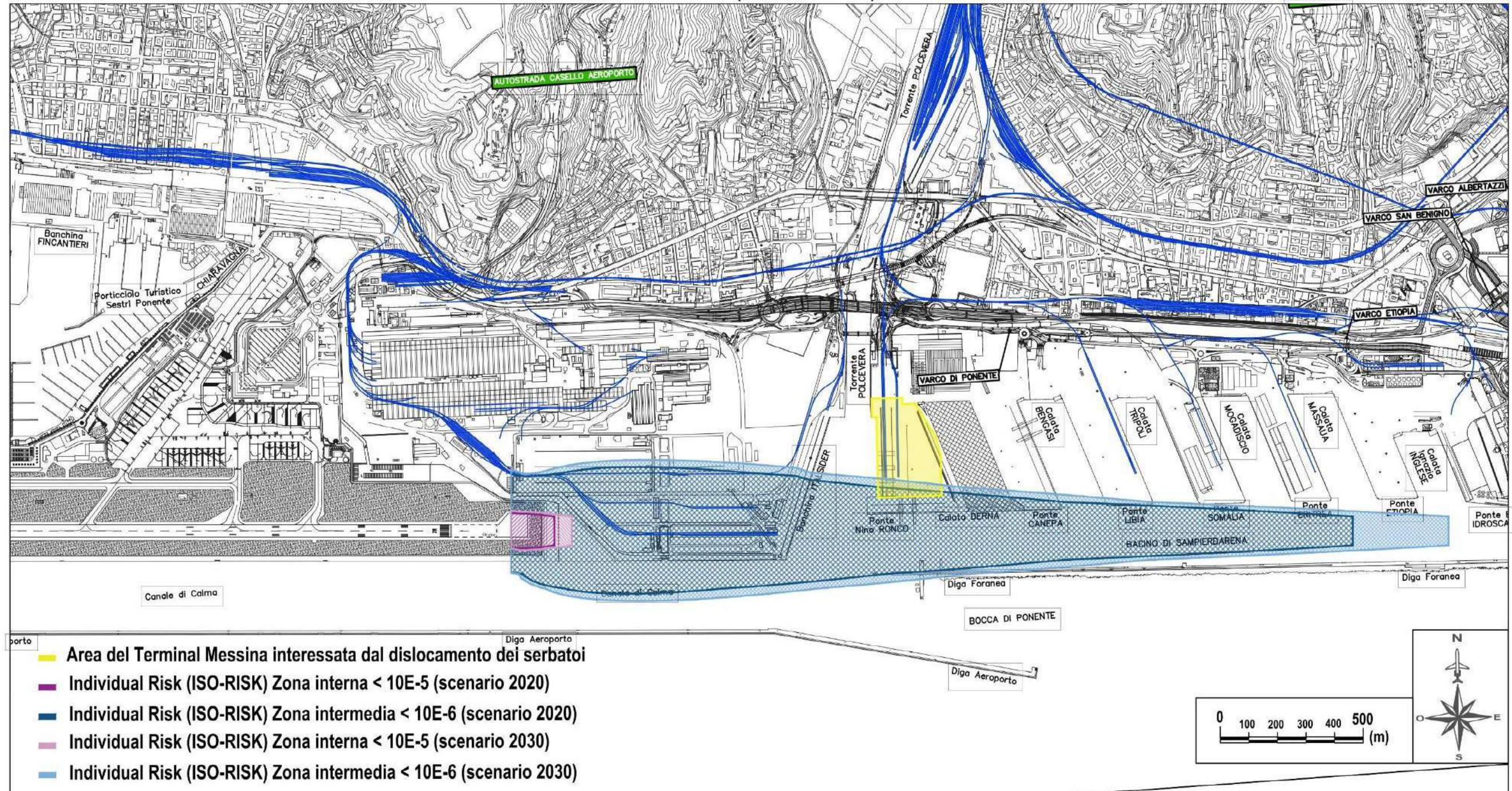
Figura 5.12. Comparazione delle curve di isorischio per gli scenari 2020 e 2030 (Testata RWY 28)
