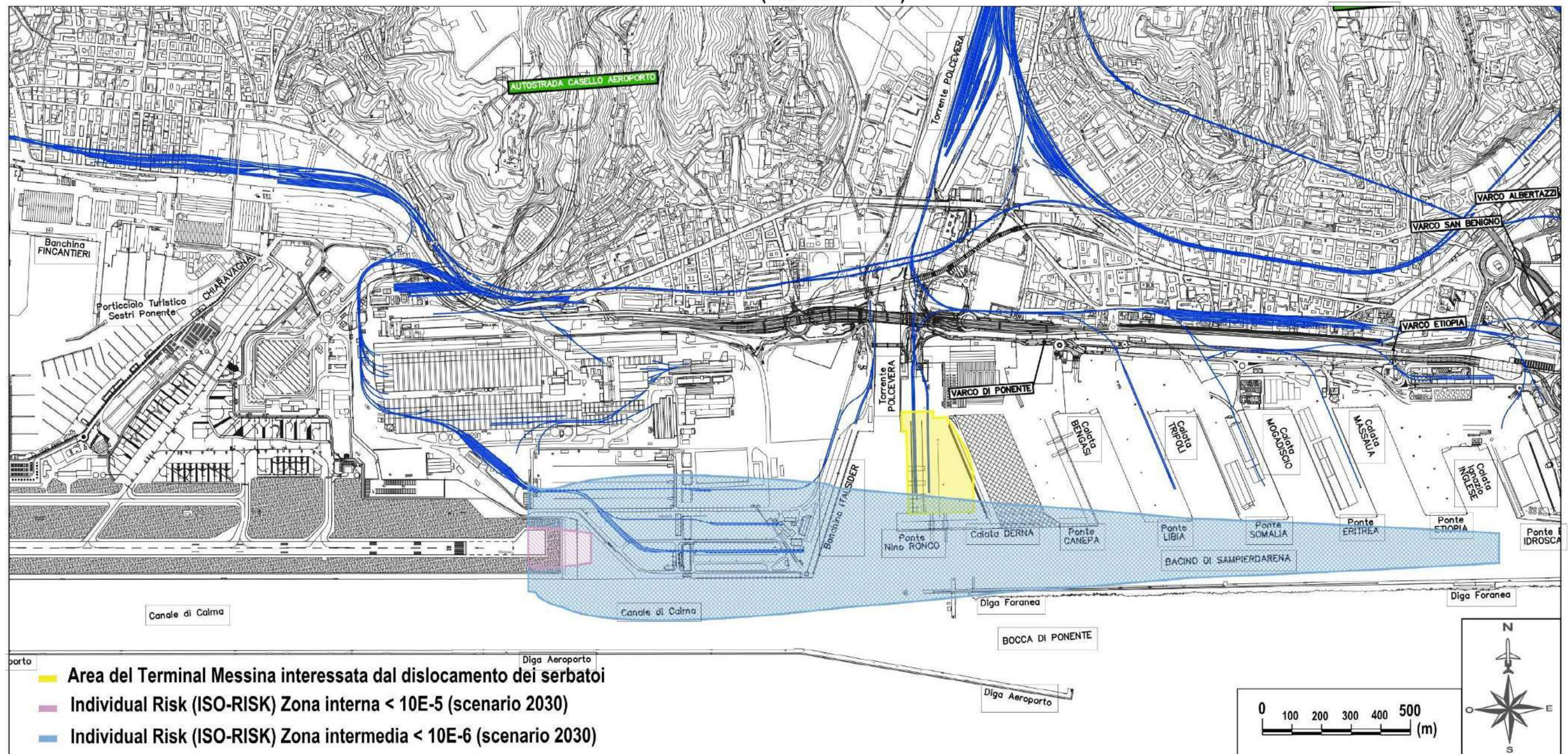
Figura 5.10. Valutazione del Rischio Contro Terzi - Scenario 2030 (Testata RWY28)
