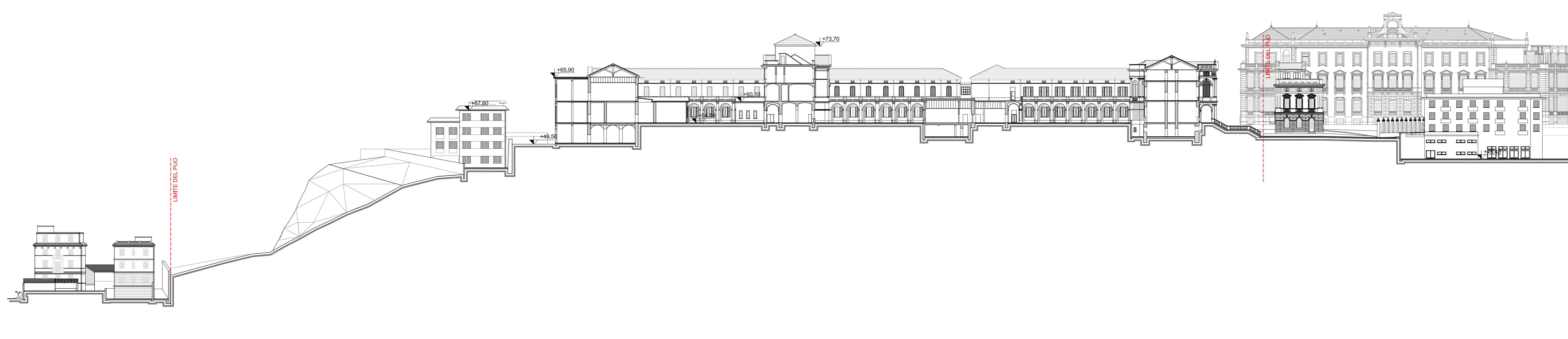
SEZIONE A-A'
