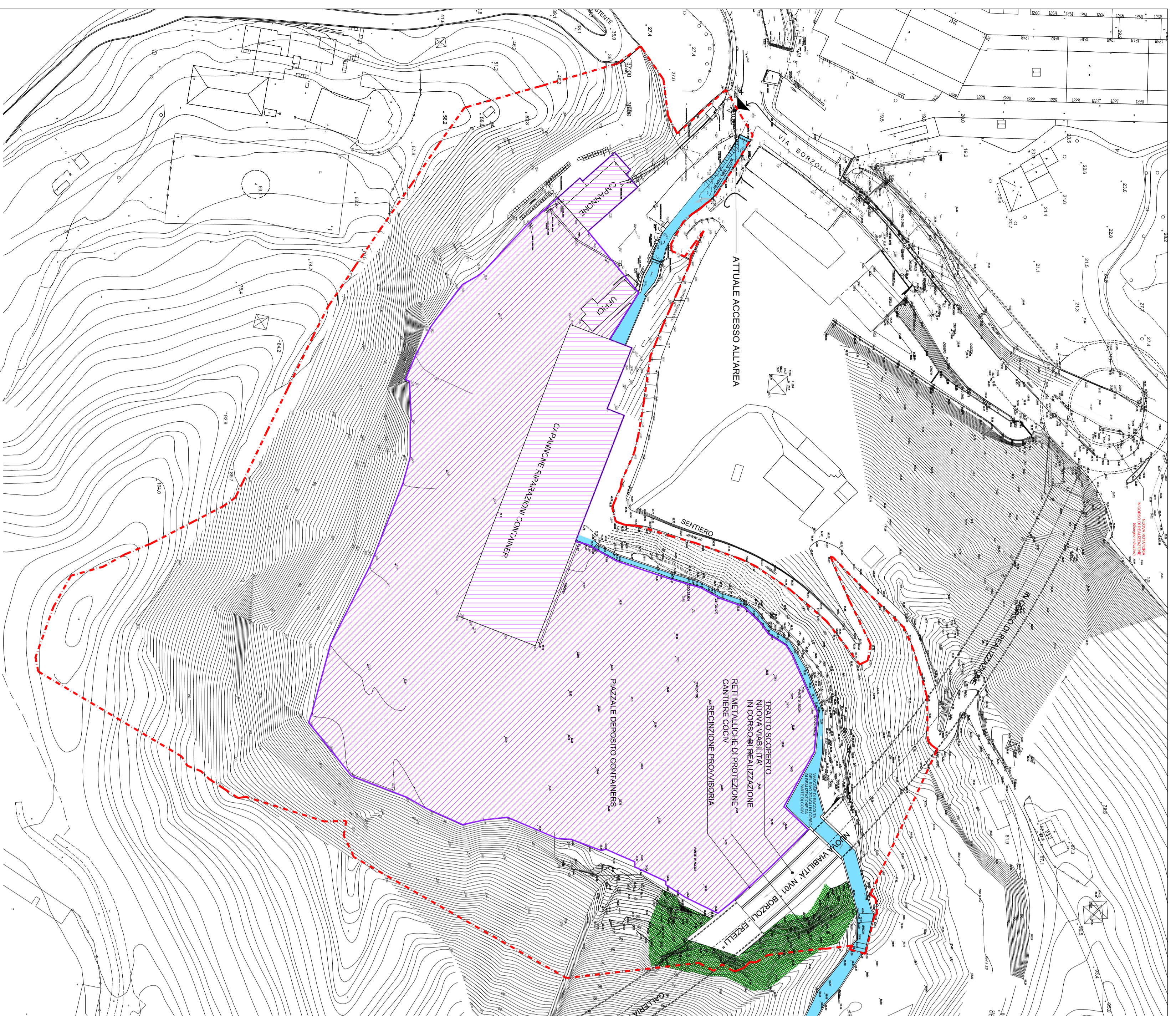
Planimetria rilievo stato attuale piazzale container 1/10000
