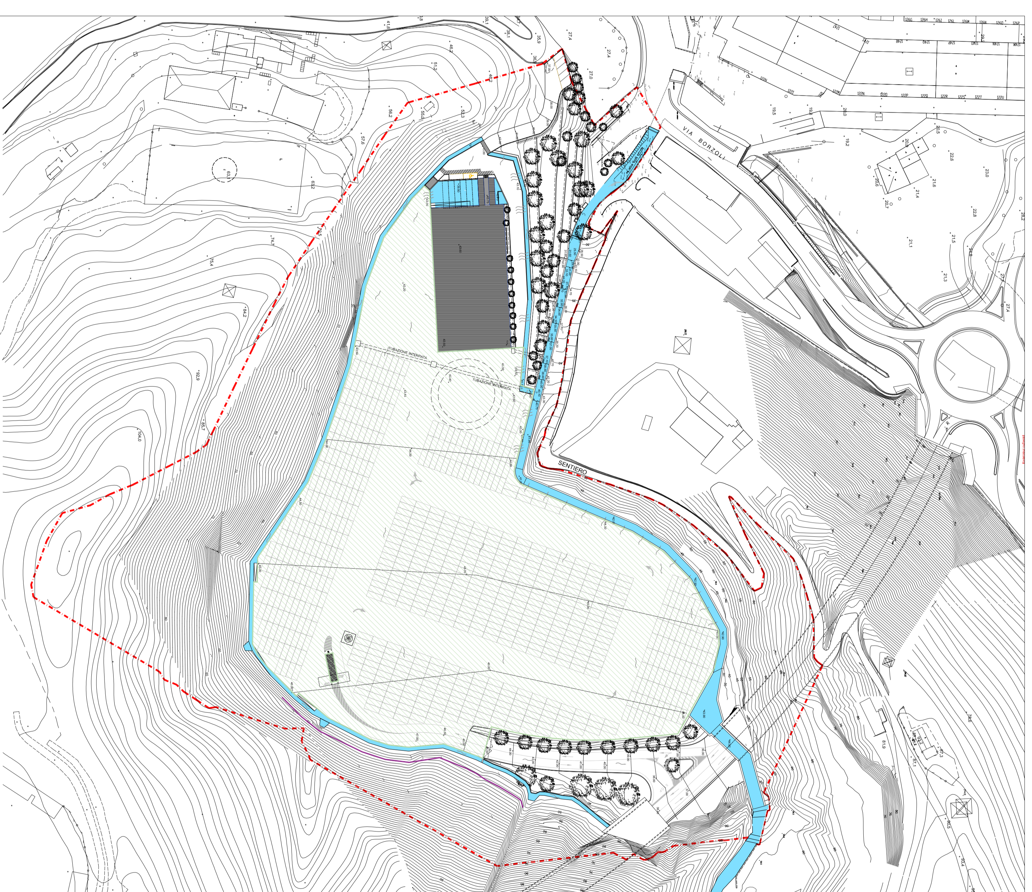
Planimetria di progetto piazzale container 1/10000
