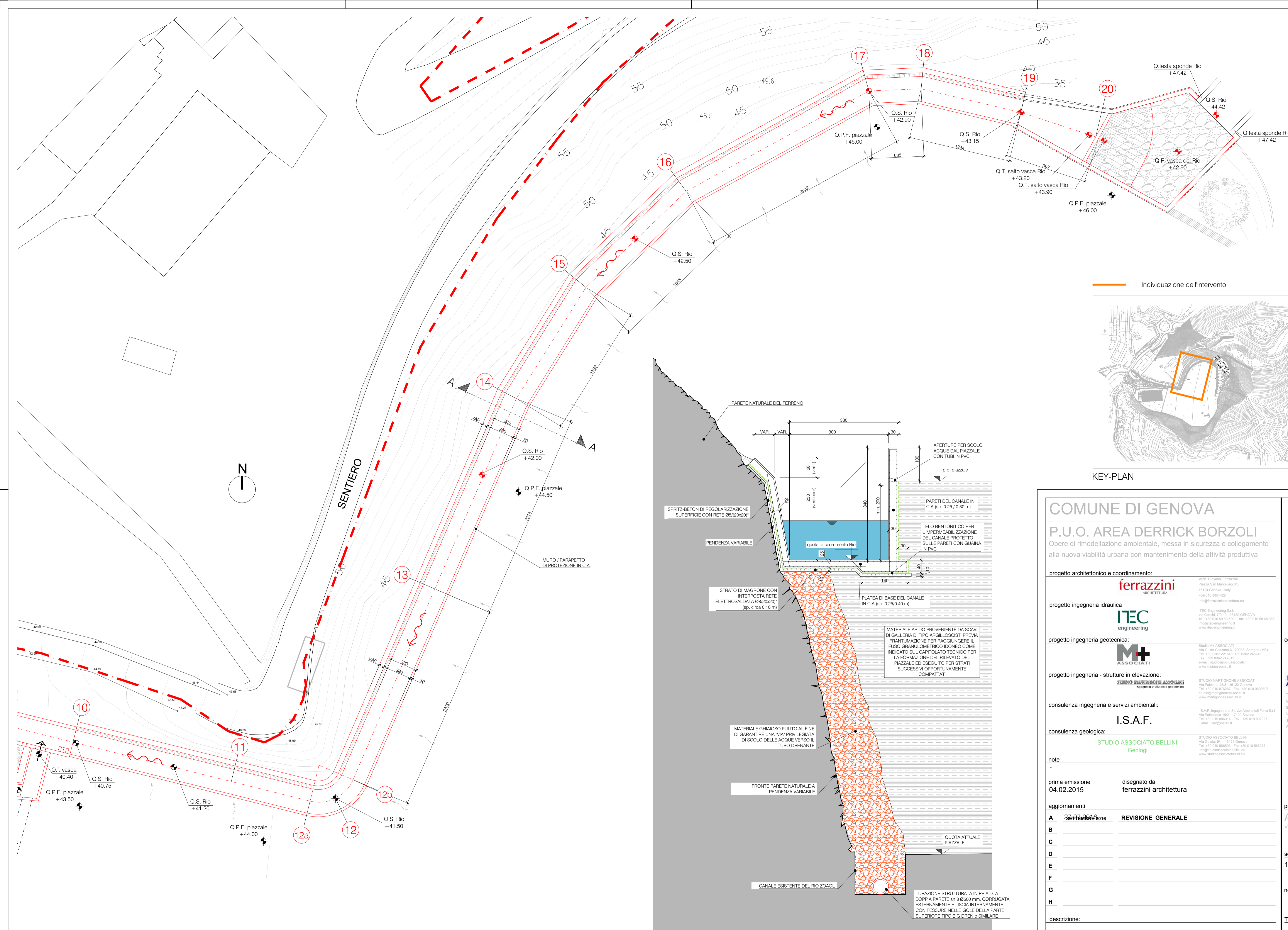
SEZIONE TIPO A - A SCALA 1:50
